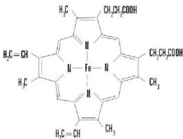
Obr. 16: Chemická struktura hemu [převzato z http://sciaga.onet.pl/20096,1,sciaga_druk.html , staženo 15.6.2010]
