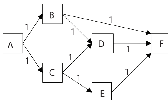
Obr. 8.6: Príklad grafu s nejednoznačnou synchronizáciou
