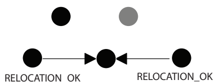
Obr. 8.9: Potvrdenie výzvy
