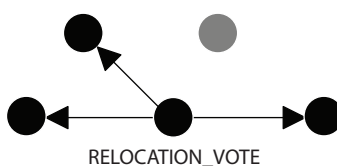
Obr. 8.8: Začiatok hlasovania
