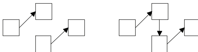
Obr. 5.1: Spojovanie podgrafov
