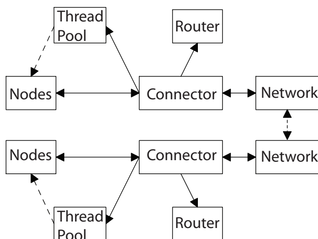
Obr. 3.1: Moduly aplikácie
