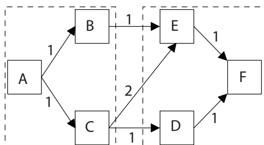
Obr. 4.1: Distribuovaný stavový automat
