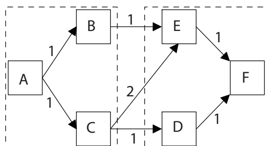
Obr. 2.1: Distribuovaný stavový automat
