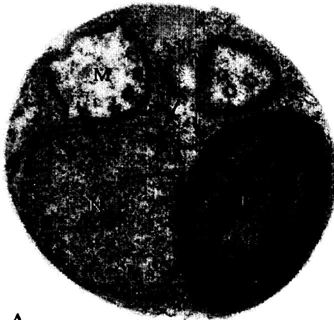
A Obr. 3: ultrastruktura Nannochloropsis oculata , zřetelně viditelný jediný plastid a mitochondrie, P-plastid, N-jádro, M-mitochondrie, vnější membrána jádra (dlouhá šipka) a povrchová membrána plastidu (krátká šipka) jsou spojené a tvoří kontinuum, měřítko= 200 nm (Murakami et al., 2009)
