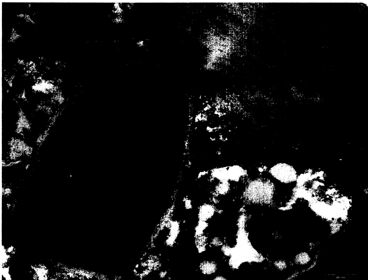
Obr. 20: E4f, polygonální pyrenoid na stopce vycházející z chloroplastu
