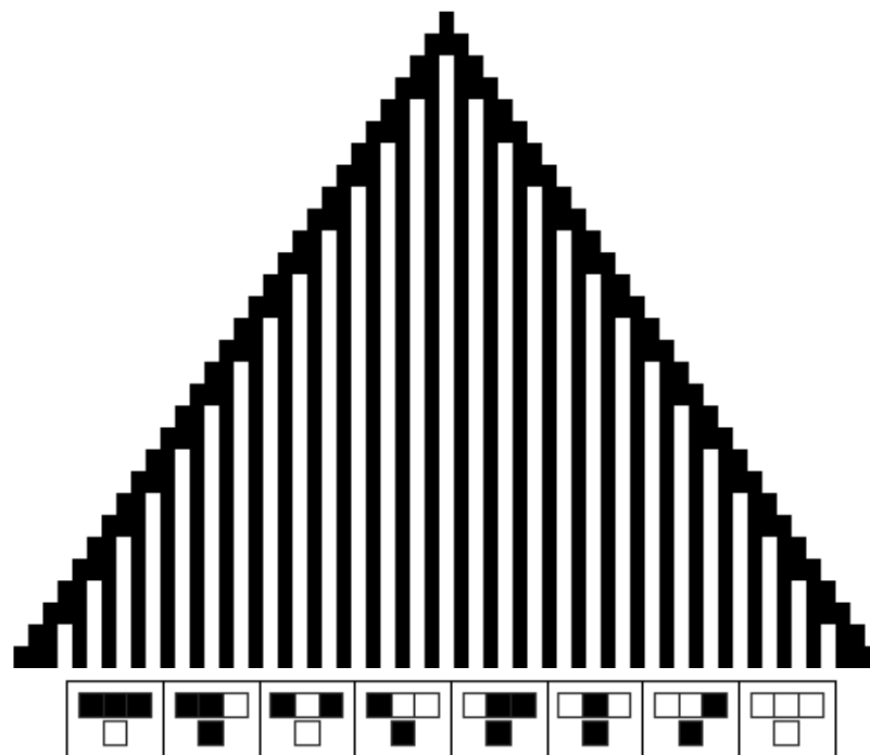
Obrázek 1.2: Elementární automat číslo 94
