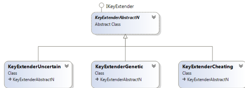
Obrázek 4.1: KeyExtenderAbstractN
