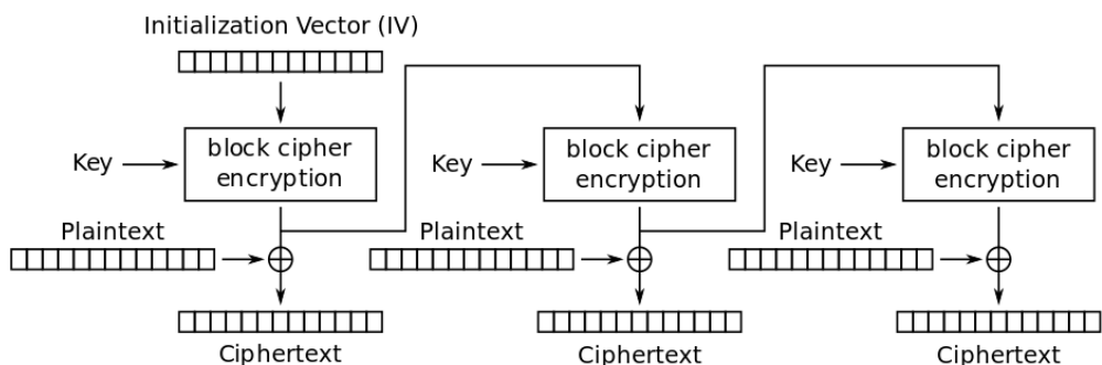
Obrázek 2.7: OFB encryption
