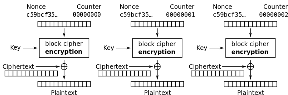
Obrázek 2.10: CTR decryption
