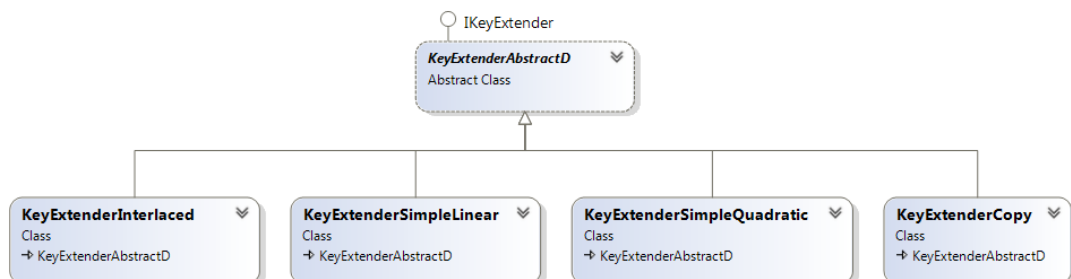
Obrázek 4.2: KeyExtenderAbstractD
