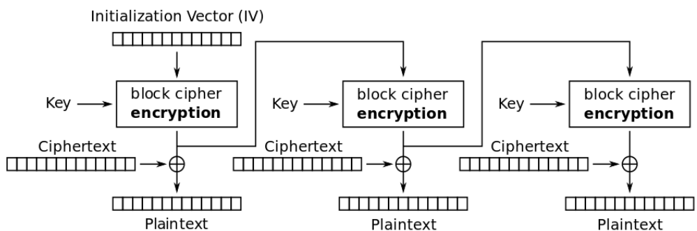
Obrázek 2.8: OFB decryption
