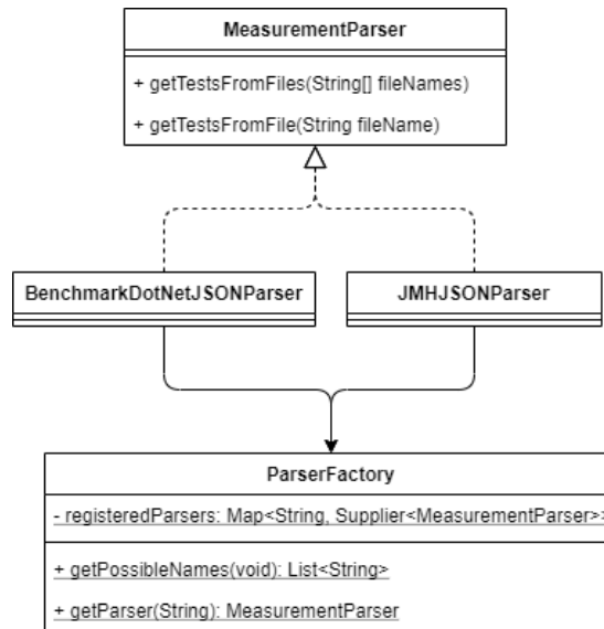
Obrázek 5.1: Struktura části PerfEvalu - návrhový vzor factory
