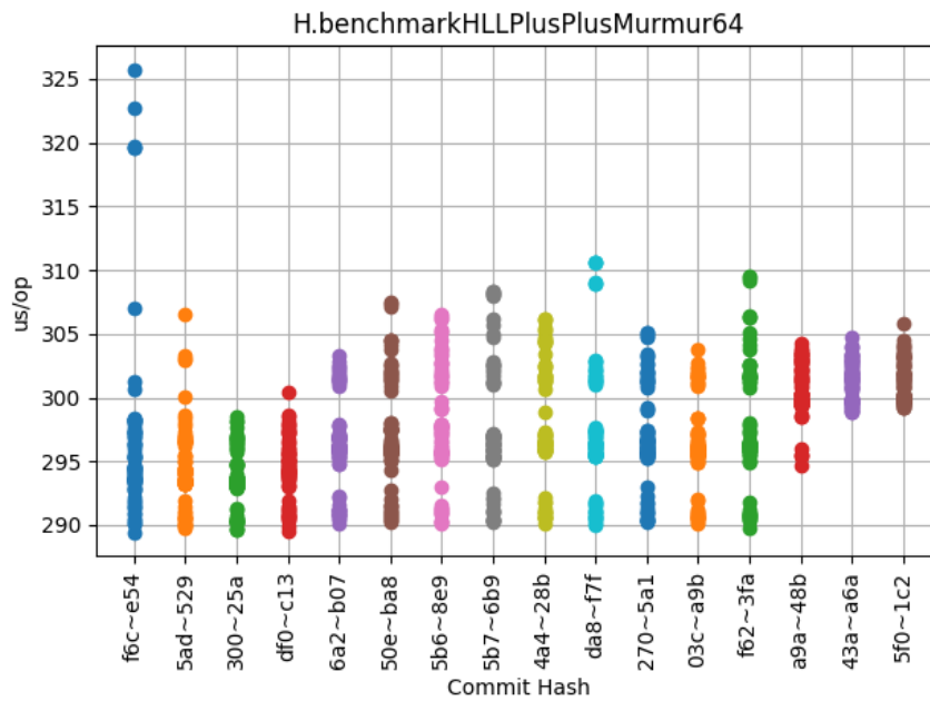
Obrázek 6.36: H.benchmarkHLLPlusPlusMurmur64
