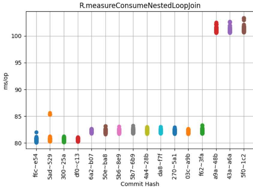
Obrázek 6.14: R.measureConsumeNestedLoopJoin
