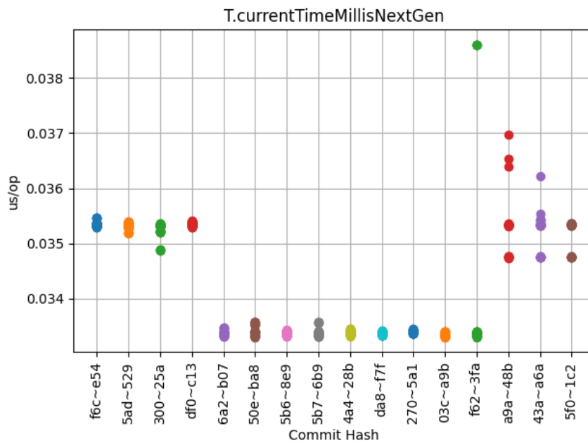
Obrázek 6.24: T.currentTimeMillisNextGen
