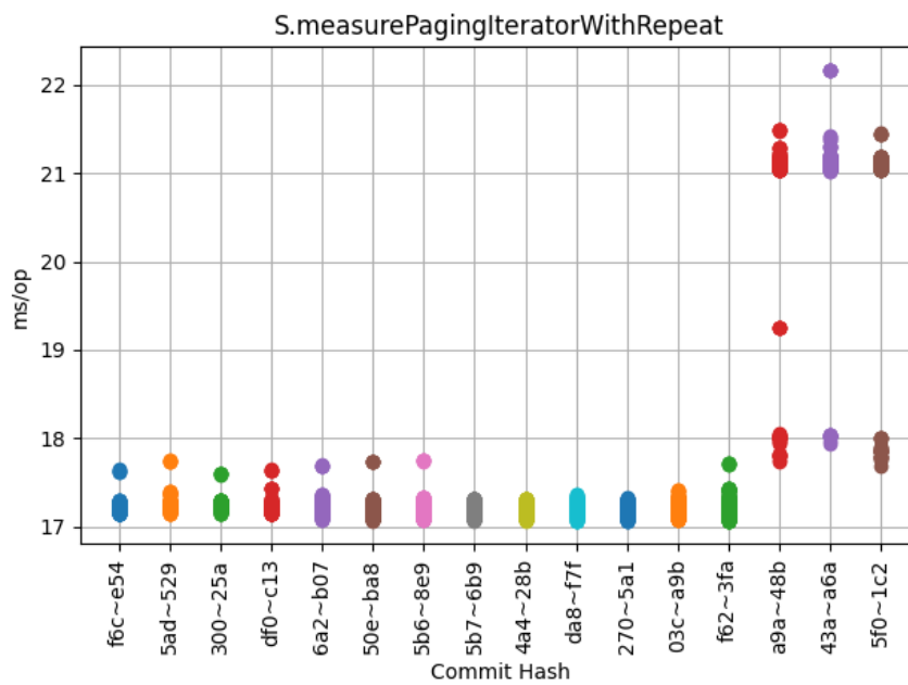
Obrázek 6.18: S.measurePagingIteratorWithRepeat
