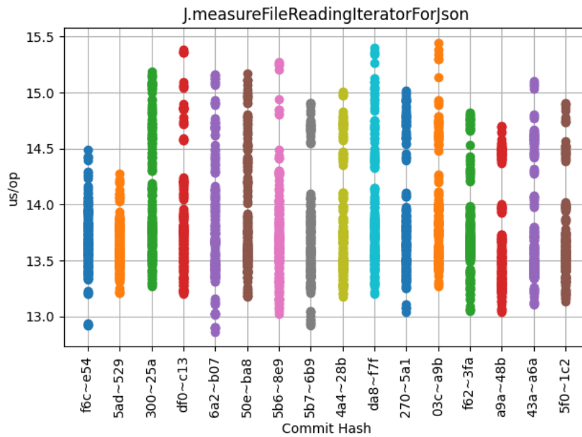
Obrázek 6.38: J.measureFileReadingIteratorForJson
