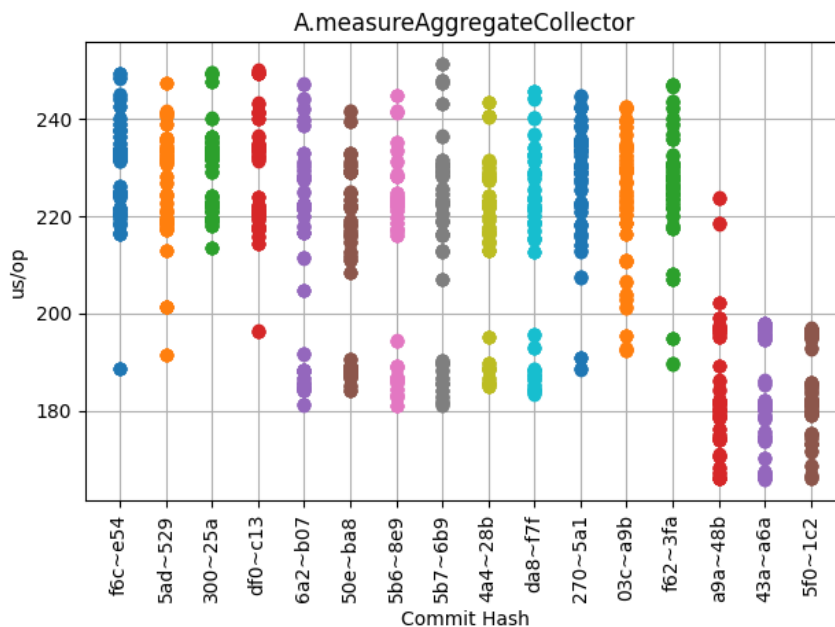
Obrázek 6.2: A.measureAggregateCollector
