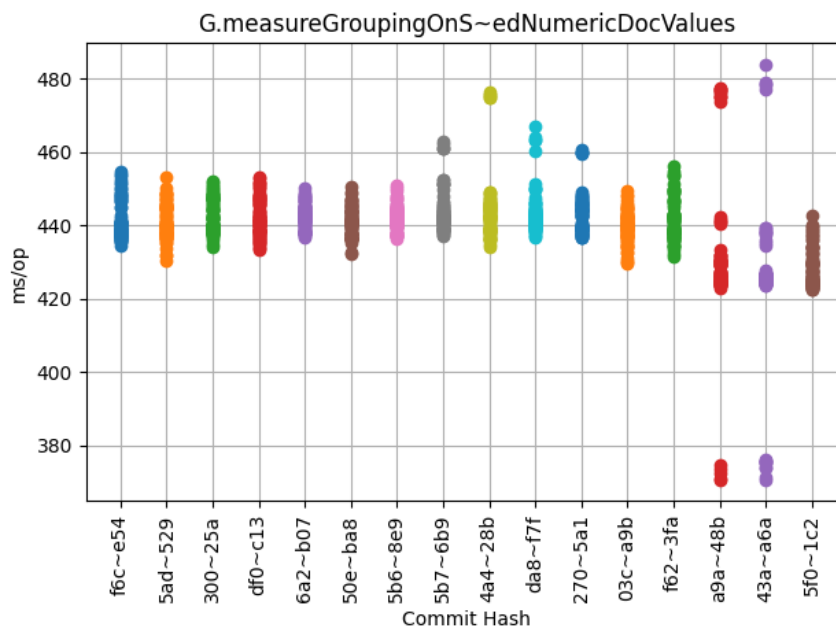
Obrázek 6.32: G.measureGroupingOnS~edNumericDocValues
