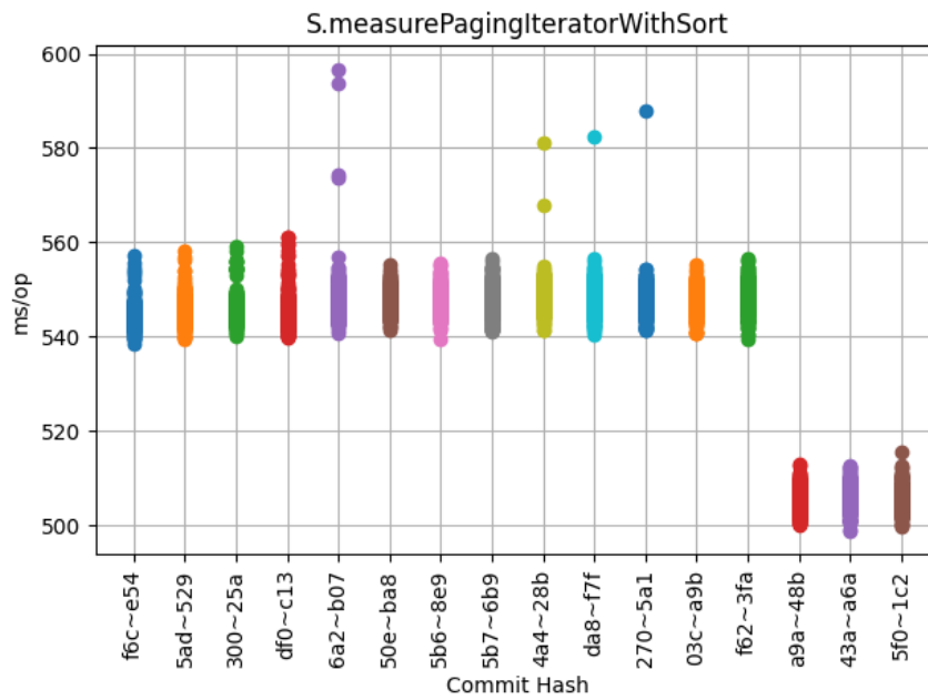
Obrázek 6.19: S.measurePagingIteratorWithSort
