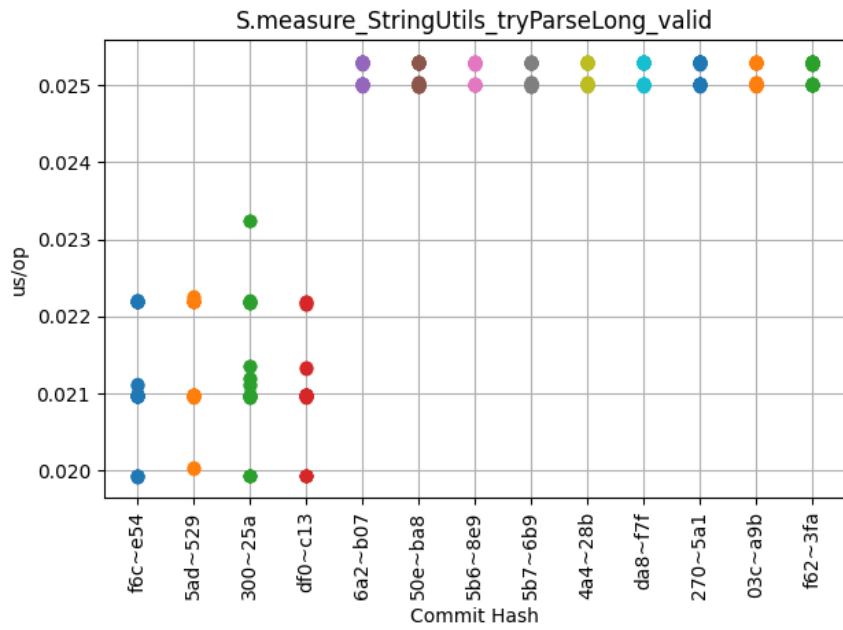
Obrázek 6.22: S.measure_StringUtils_tryParseLong_valid
