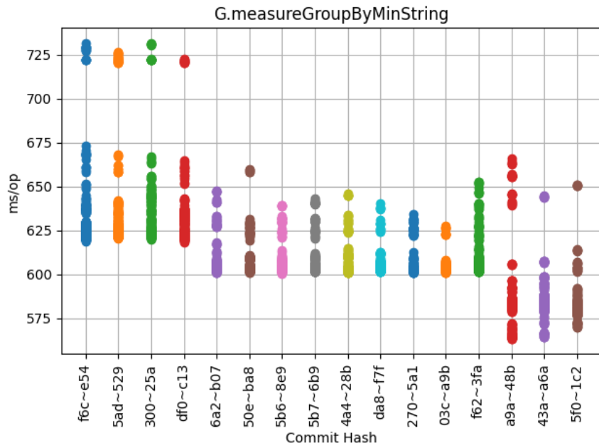
Obrázek 6.28: G.measureGroupByMinString
