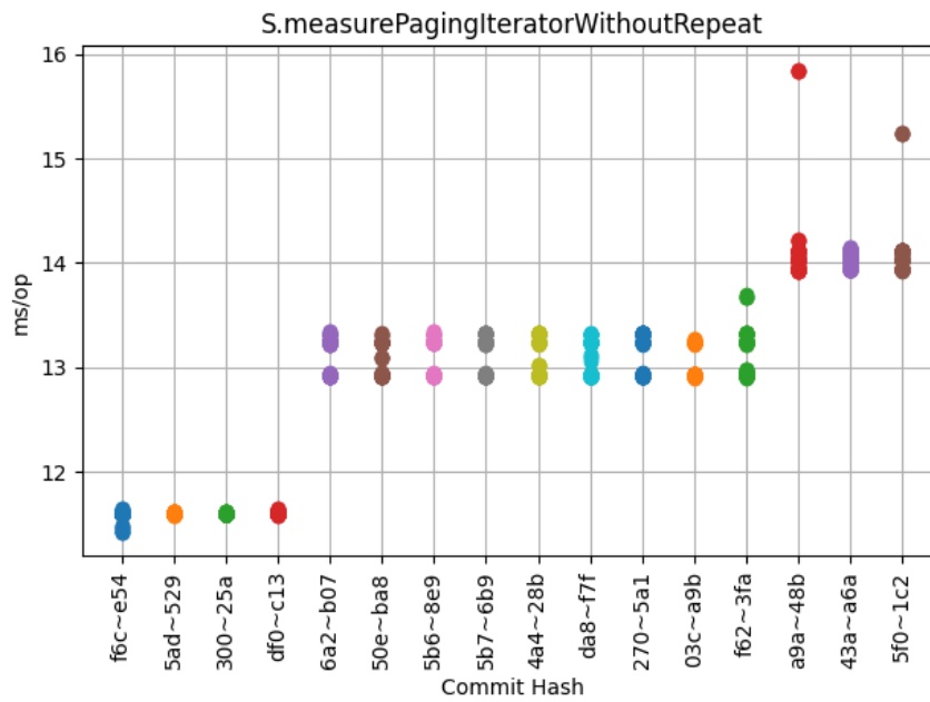
Obrázek 6.17: S.measurePagingIteratorWithoutRepeat
