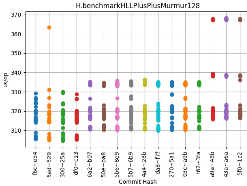
Obrázek 6.35: H.benchmarkHLLPlusPlusMurmur128
