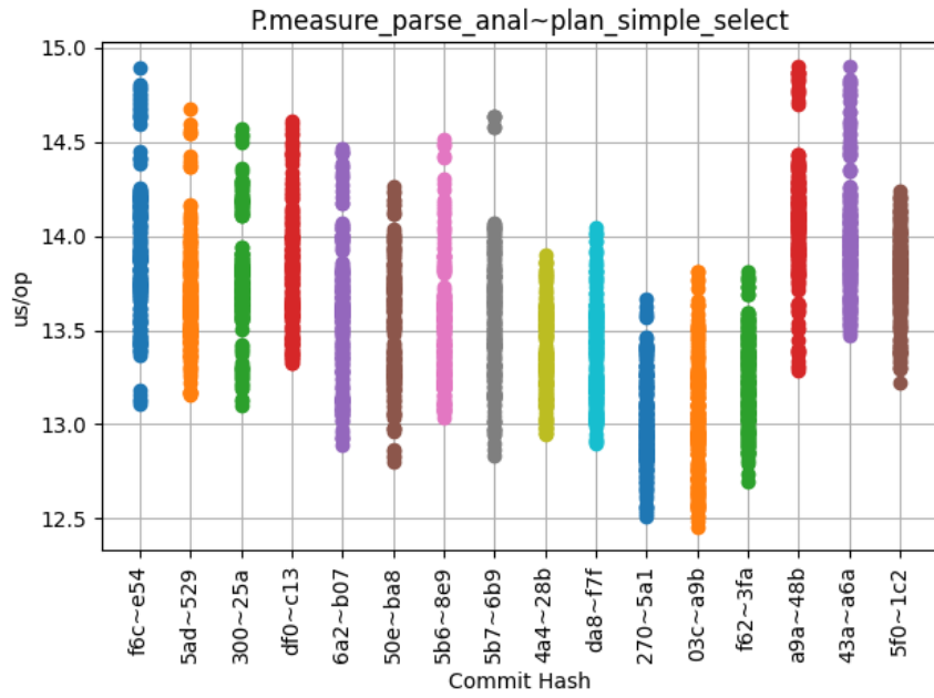
Obrázek 6.8: P.measure_parse_anal~plan_simple_select
