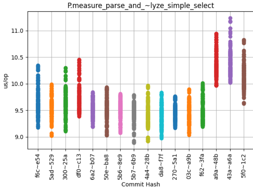
Obrázek 6.9: P.measure_parse_and_~lyze_simple_select
