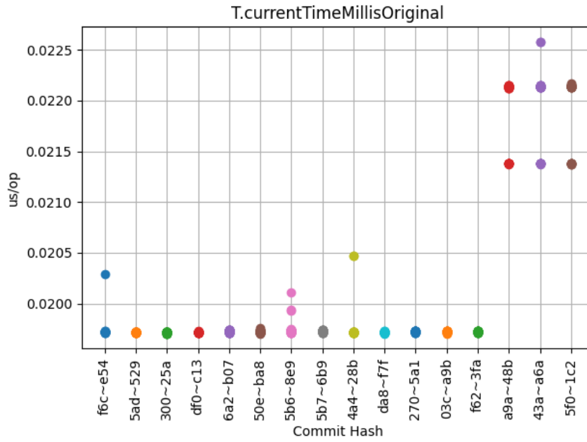
Obrázek 6.25: T.currentTimeMillisOriginal
