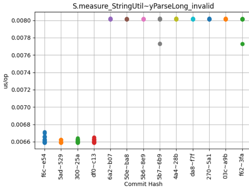
Obrázek 6.23: S.measure_StringUtil~yParseLong_invalid
