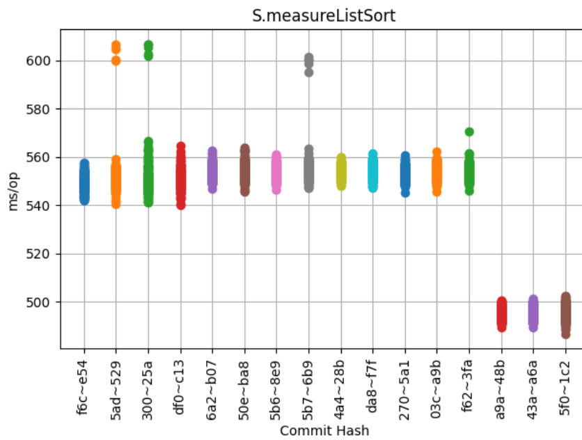
Obrázek 6.16: S.measureListSort
