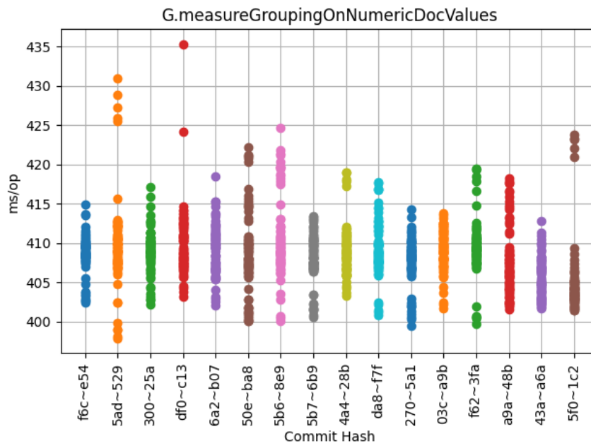
Obrázek 6.31: G.measureGroupingOnNumericDocValues
