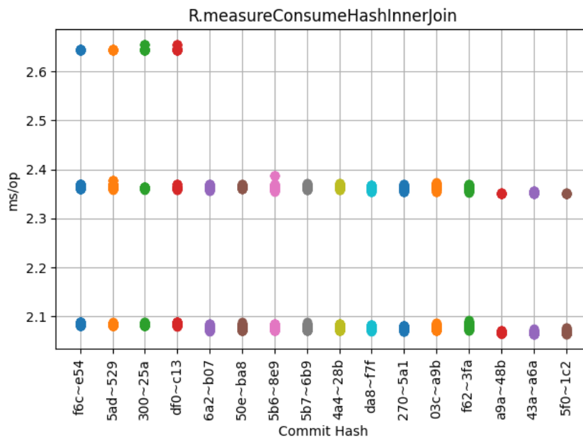
Obrázek 6.12: R.measureConsumeHashInnerJoin
