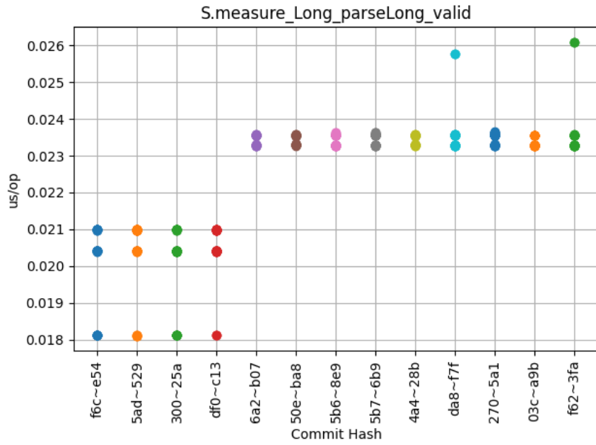
Obrázek 6.21: S.measure_Long_parseLong_valid
