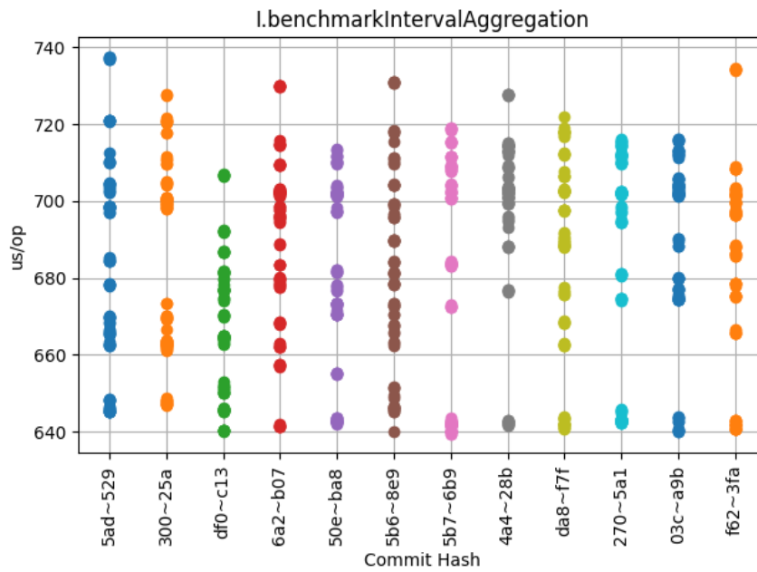
Obrázek 6.37: I.benchmarkIntervalAggregation
