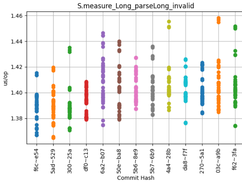
Obrázek 6.20: S.measure_Long_parseLong_invalid
