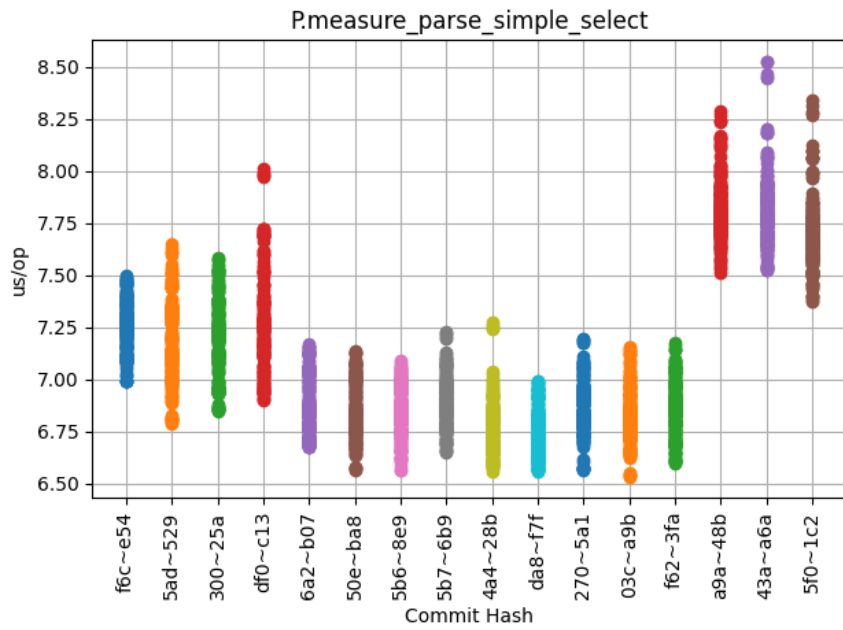
Obrázek 6.10: P.measure_parse_simple_select
