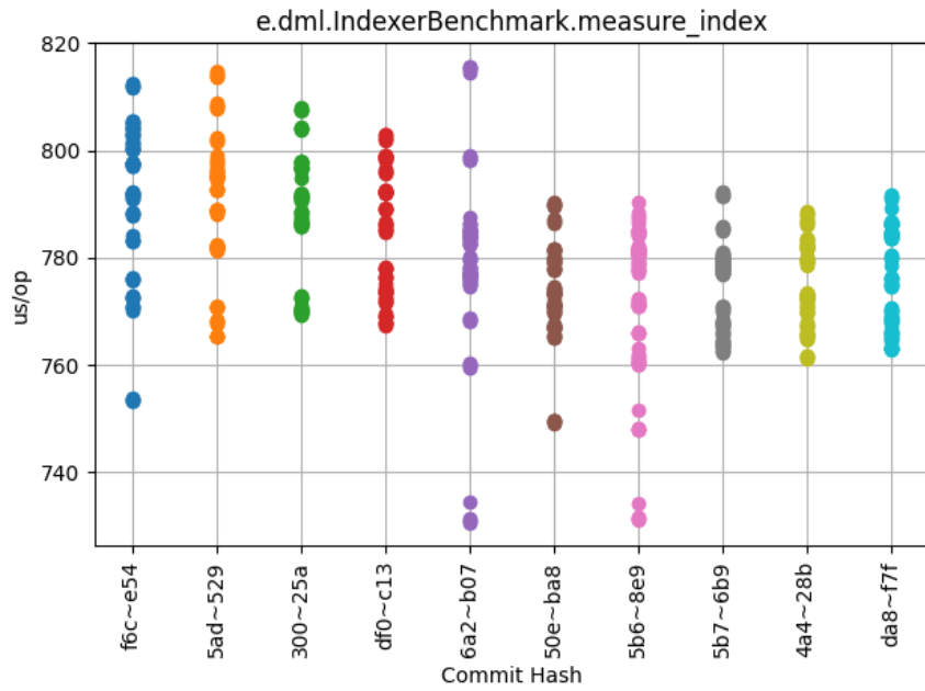
Obrázek 6.27: e.dml.IndexerBenchmark.measure_index
