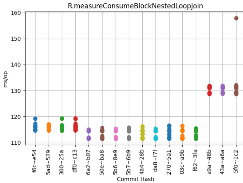
Obrázek 6.11: R.measureConsumeBlockNestedLoopJoin
