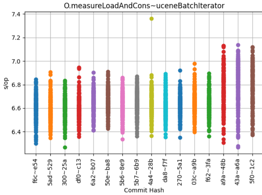
Obrázek 6.7: O.measureLoadAndCons~uceneBatchIterator
