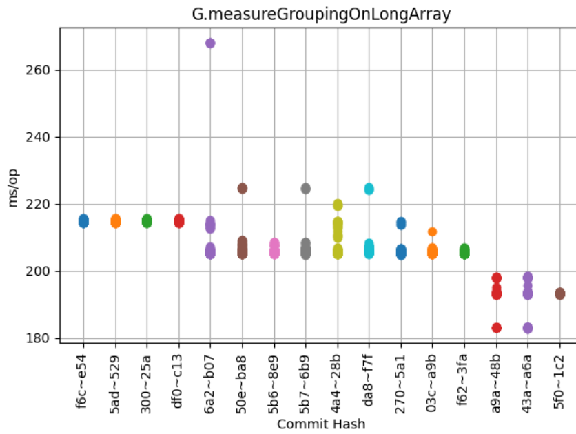
Obrázek 6.30: G.measureGroupingOnLongArray
