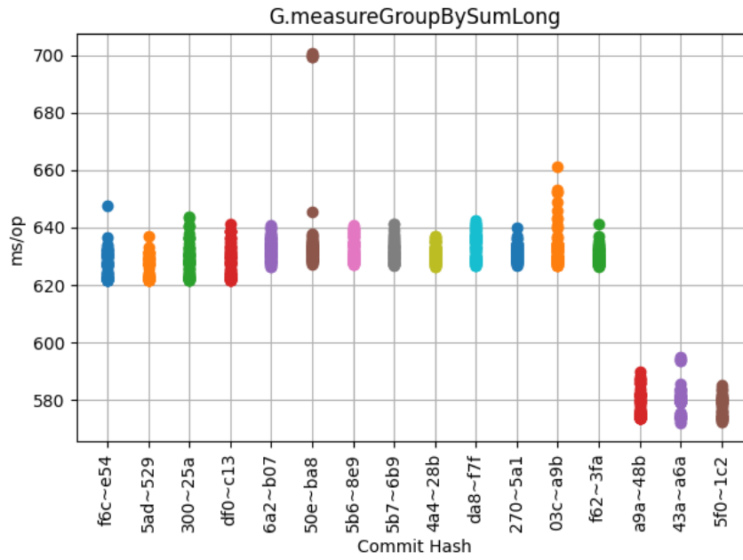
Obrázek 6.29: G.measureGroupBySumLong
