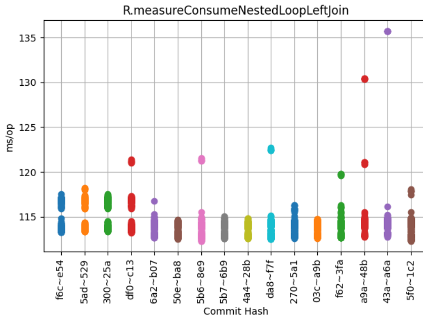
Obrázek 6.15: R.measureConsumeNestedLoopLeftJoin
