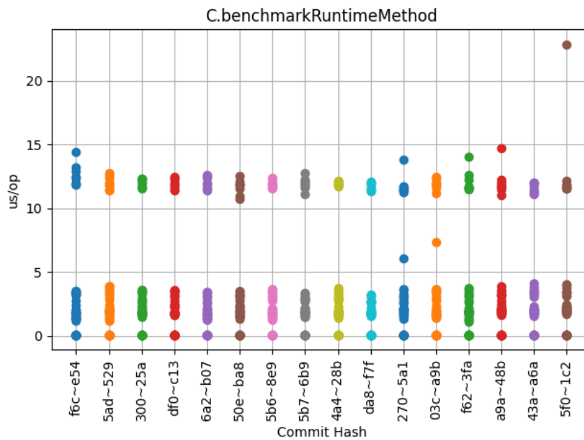
Obrázek 6.4: C.benchmarkRuntimeMethod
