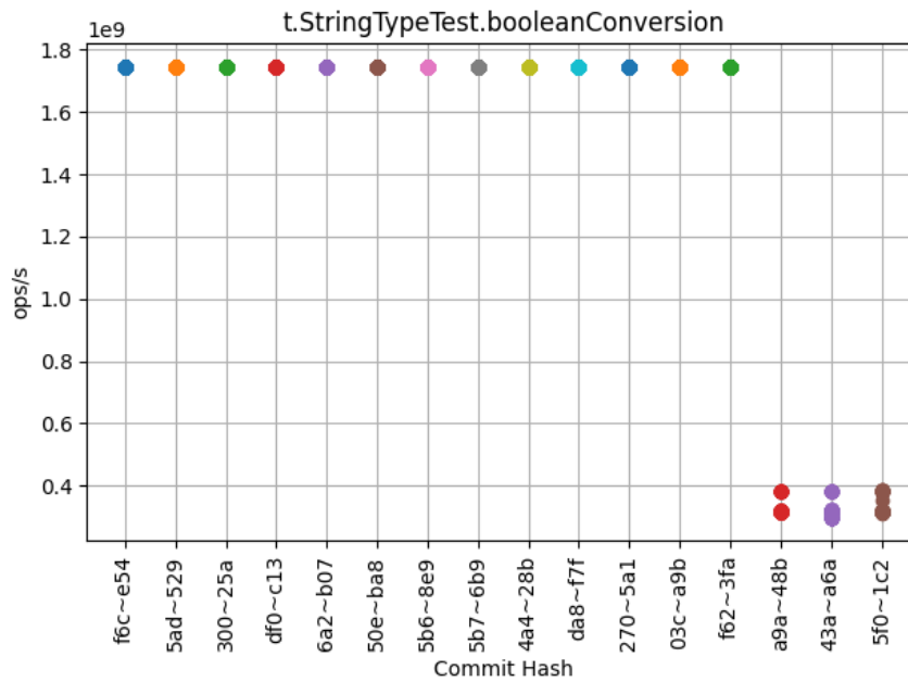
Obrázek 6.26: t.StringTypeTest.booleanConversion
