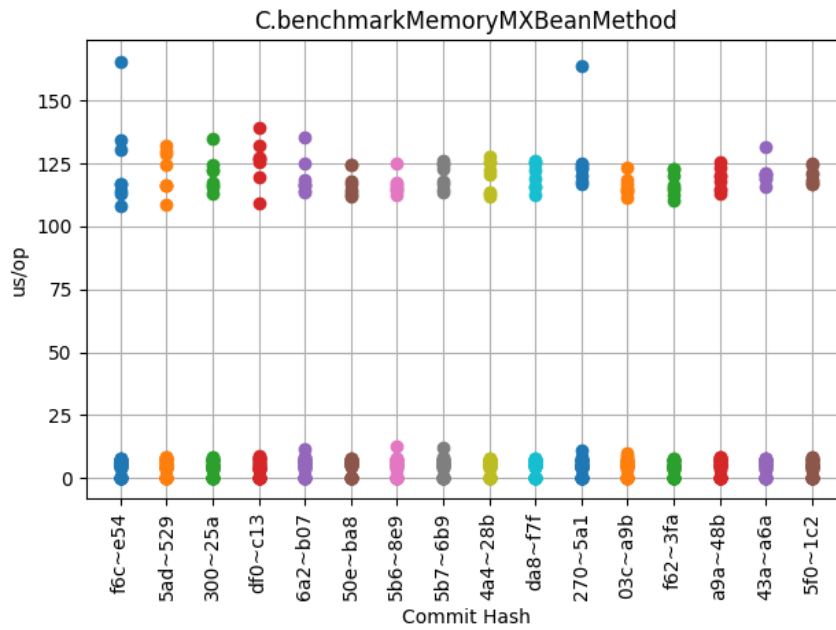
Obrázek 6.3: C.benchmarkMemoryMXBeanMethod
