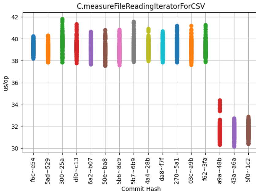
Obrázek 6.5: C.measureFileReadingIteratorForCSV
