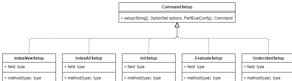
Obrázek 5.2: Struktura části PerfEvalu - návrhový vzor builder
