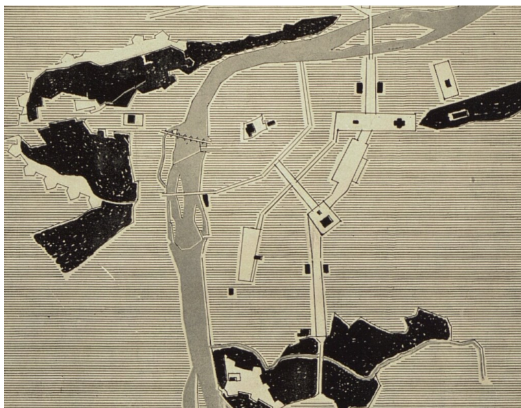
17. Koncept vedení tzv. severojižní transverzály (pozdější magistrály) v trase někdejších novoměstských hradeb se zapojením nového monumentálního náměstí Budovatelů (v místech Masarykova nádraží), 1948.
