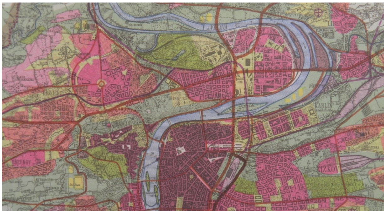
13.-14. První poválečný směrný územní plán Prahy, 1948. Rozdělení města do funkčně odlišených zón, důraz na dopravní řešení (počítáno mj. s komunikací po nábřeží Malé Strany a přes svah Petřína).
