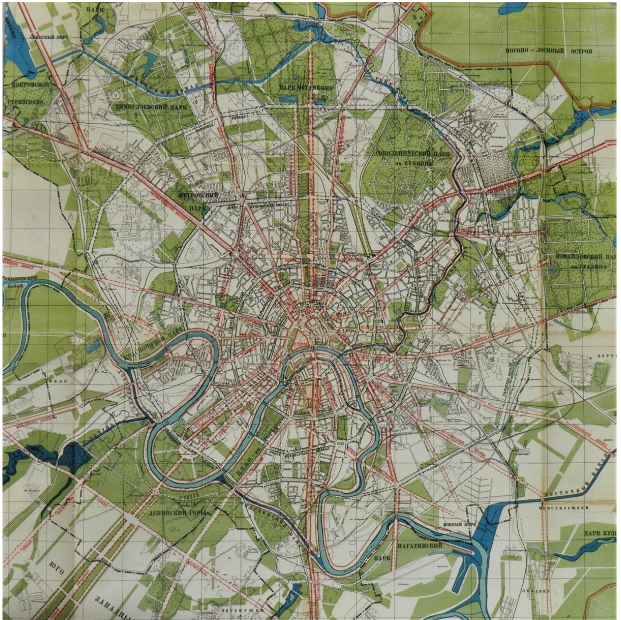
20. Generální plán Moskvy, 1935. Rozvoj města navržen v systému jednotlivých soustředných okruhů a příčných radiál vybihajících z centra. Tradiční bloková struktura nové zástavby; důraz na pravidelnost a symetrii.
