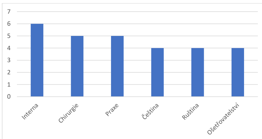
Graf 2: Maturitní předměty
