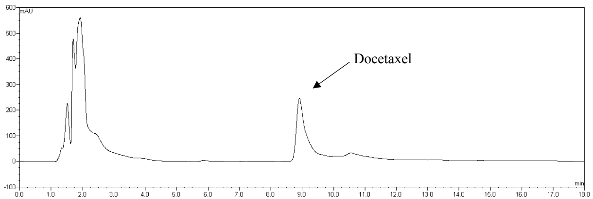
Obrázek 2 Chromatografický záznam docetaxelu.
