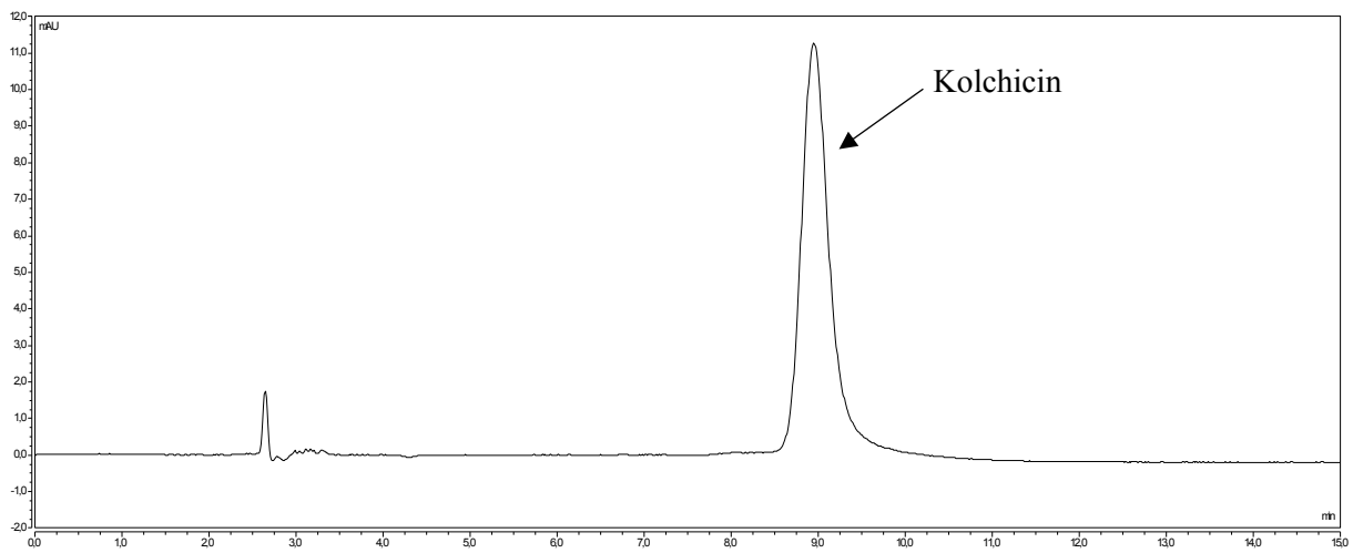
Obrázek 1 Chromatografický záznam kolchicinu.
