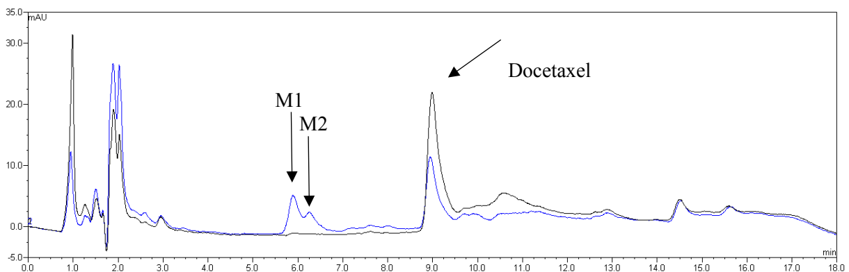
Obrázek 3 Chromatografický záznam metabolismu docetaxelu jaterními mikrosomy potkanů premedikovaných pomocí pregnenolonkarbonitrilu (modrá) v porovnání s kontrolou (bez NADPH-generujícího systému, černá).
