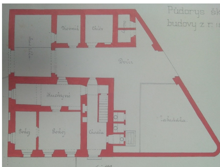
Obr.2 – půdorys přízemí první školní budovy (Kronika Obecné školy 1848-1933)
