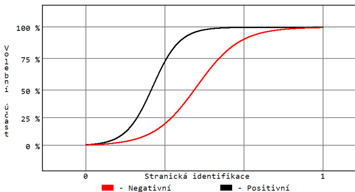
Graf 1: Logistické regresní křivky
