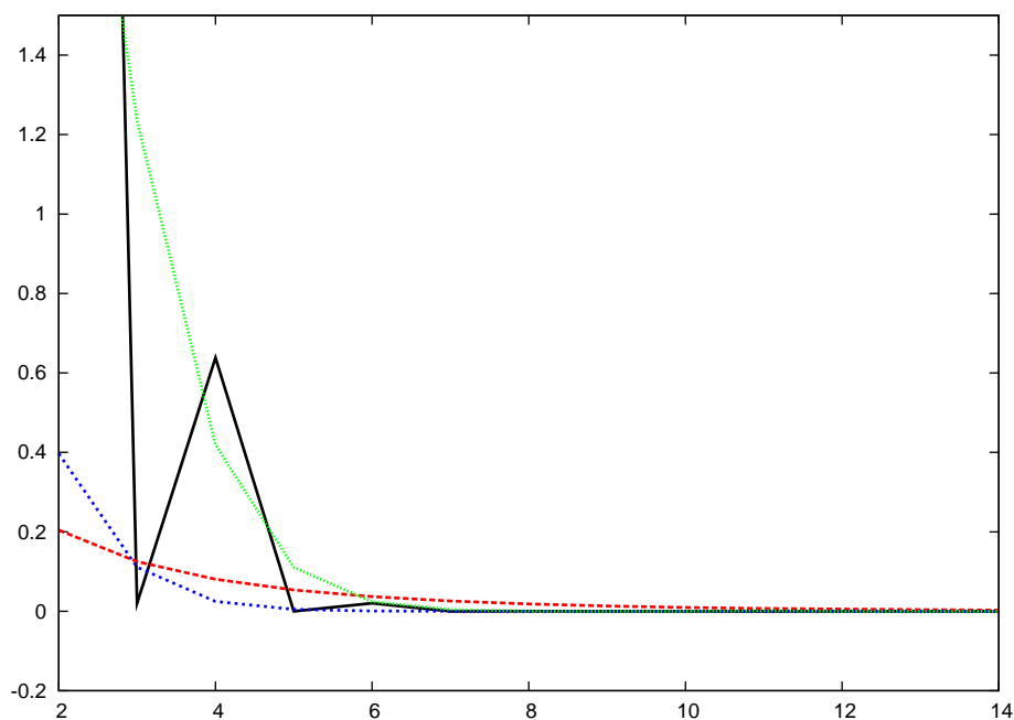
Obrázek 2: Odhady chyb pro f_3 , \varepsilon = 0.5
