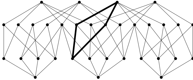
Figure 3.7. w'(bcdyz) = w'(bcdtxyz)
