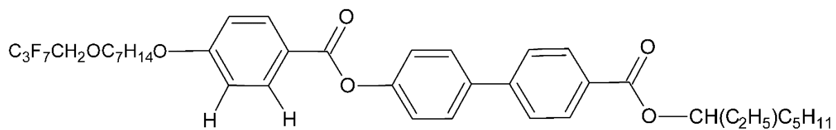
Obrázek 1 Struktury studovaných OAFLC
