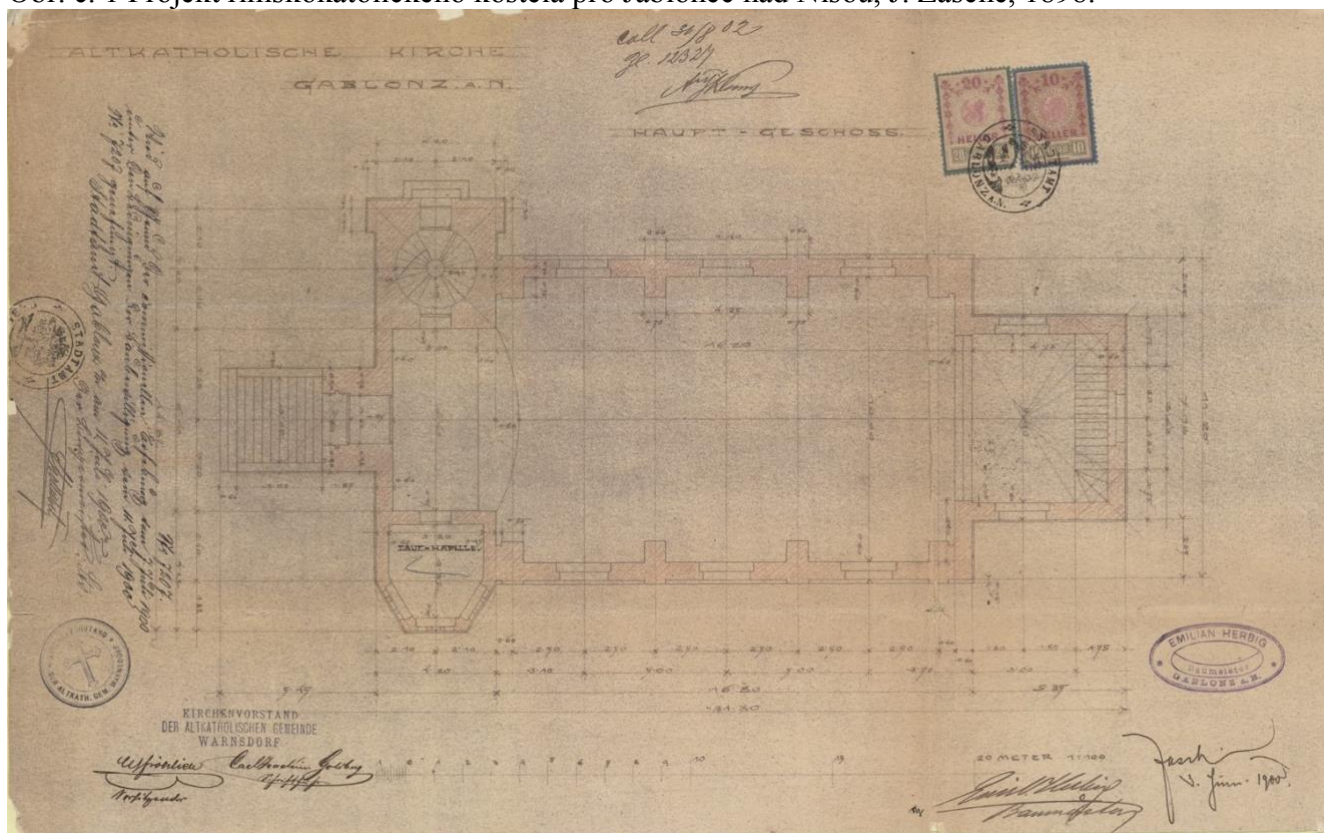
Obr. č. 2 Projekt starokatolického kostela pro Jablonec nad Nisou – plán hlavního podlaží, J. Zasche, 1900.
