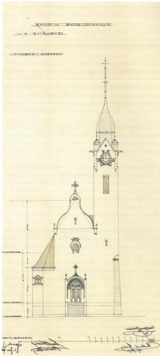
Obr. č. 3 Projekt starokatolického kostela pro Jablonec nad Nisou – průčelí s původním návrhem věže, J. Zasche, 1900.
