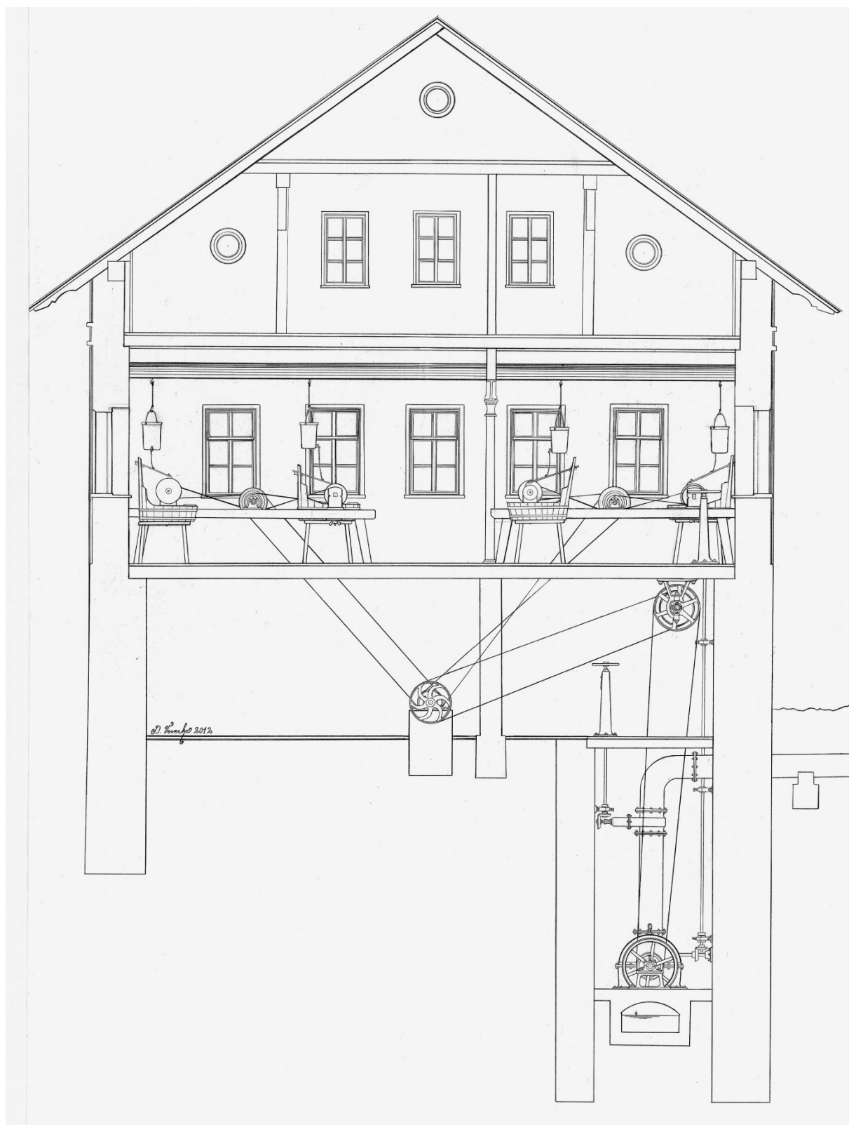
Vyobrazení brusírny skla se Schwamkrugovou turbínou, transmisními rozvody a sklářskými brusy. Kresba David Veverka.
