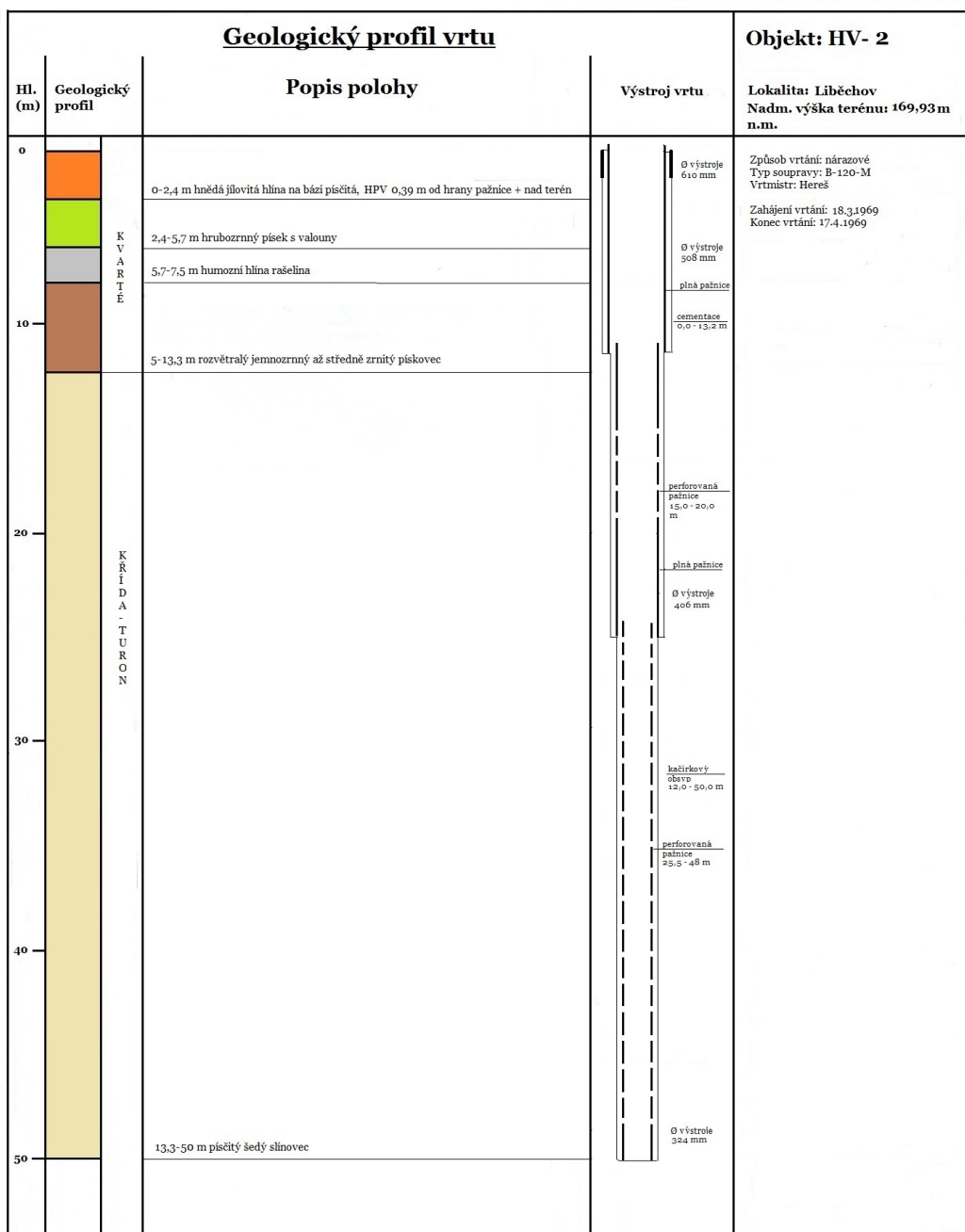
Obrázek A.2: Geologický profil vrtu HV-2
