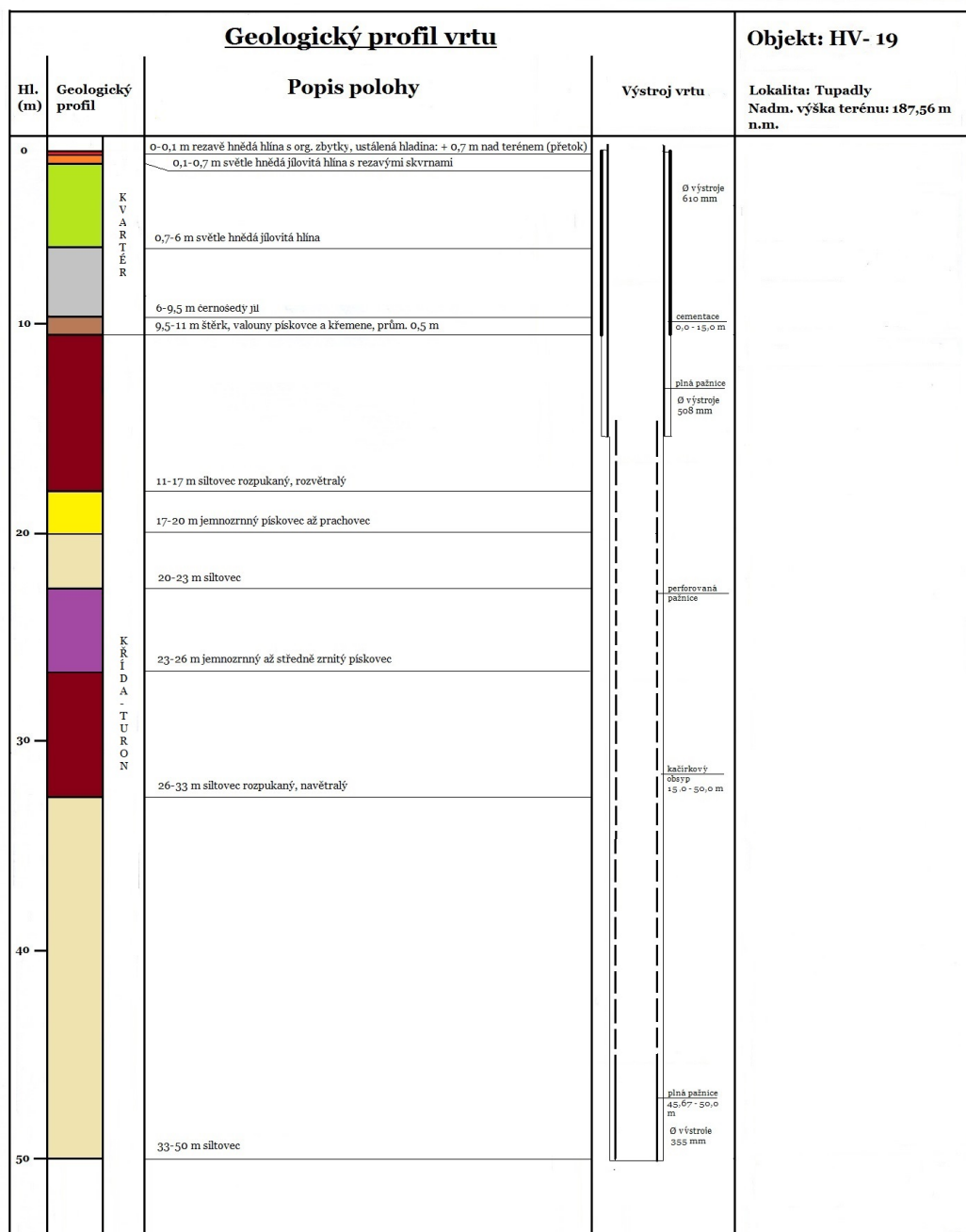
Obrázek A.3: Geologický profil vrtu HV-19
