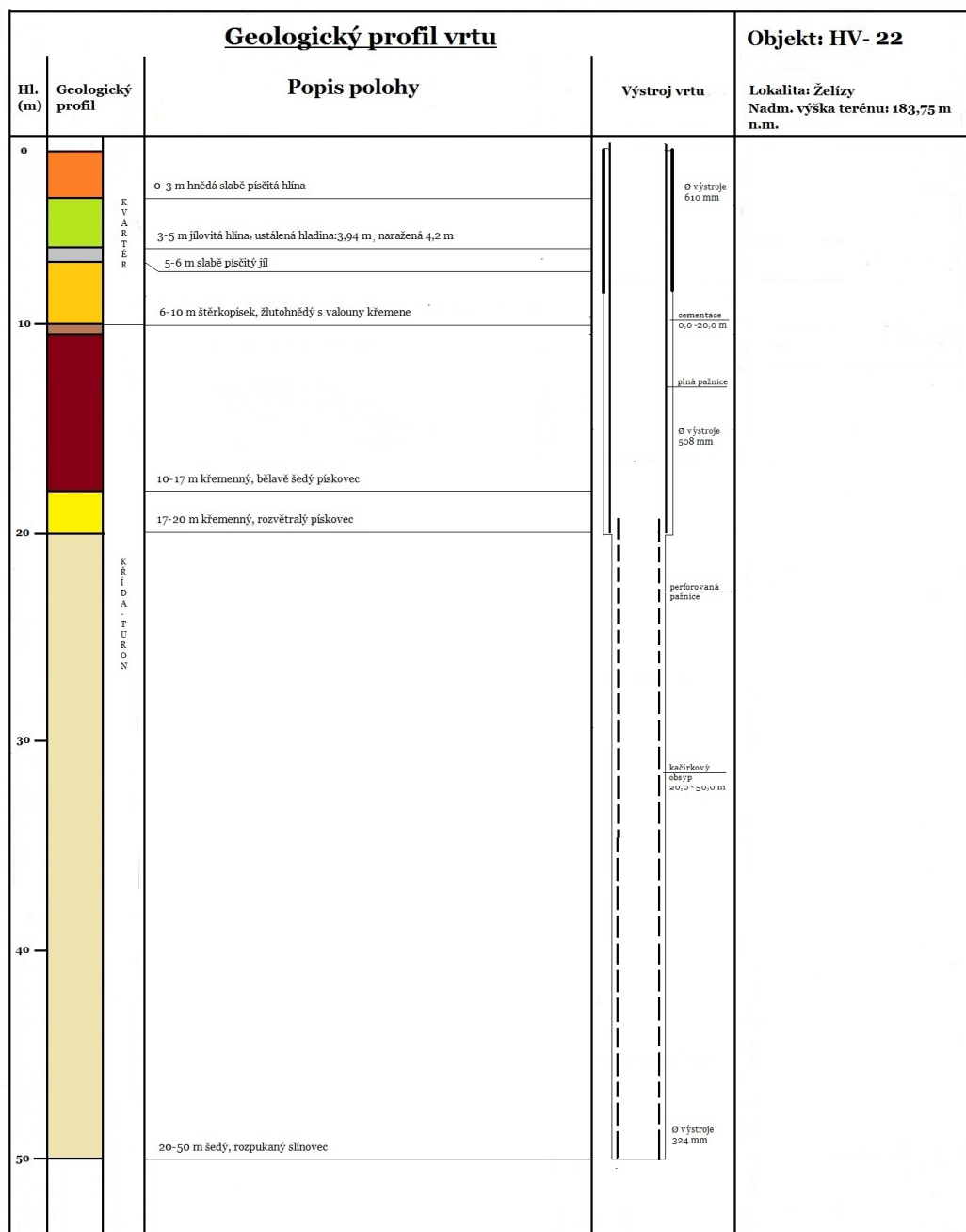
Obrázek A.4: Geologický profil vrtu HV-22
