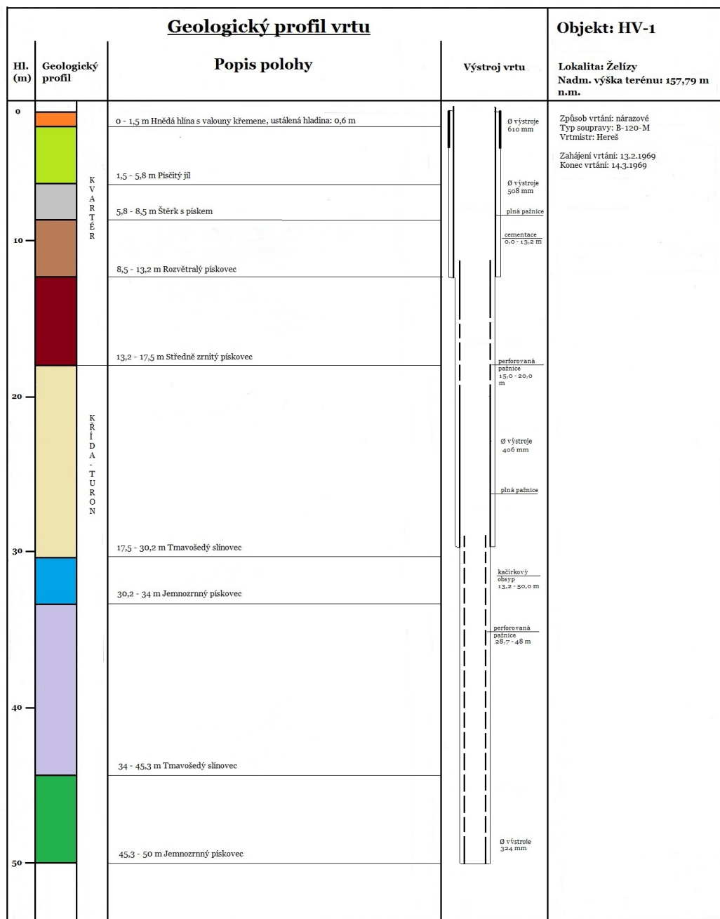
Obrázek A.1: Geologický profil vrtu HV-1
