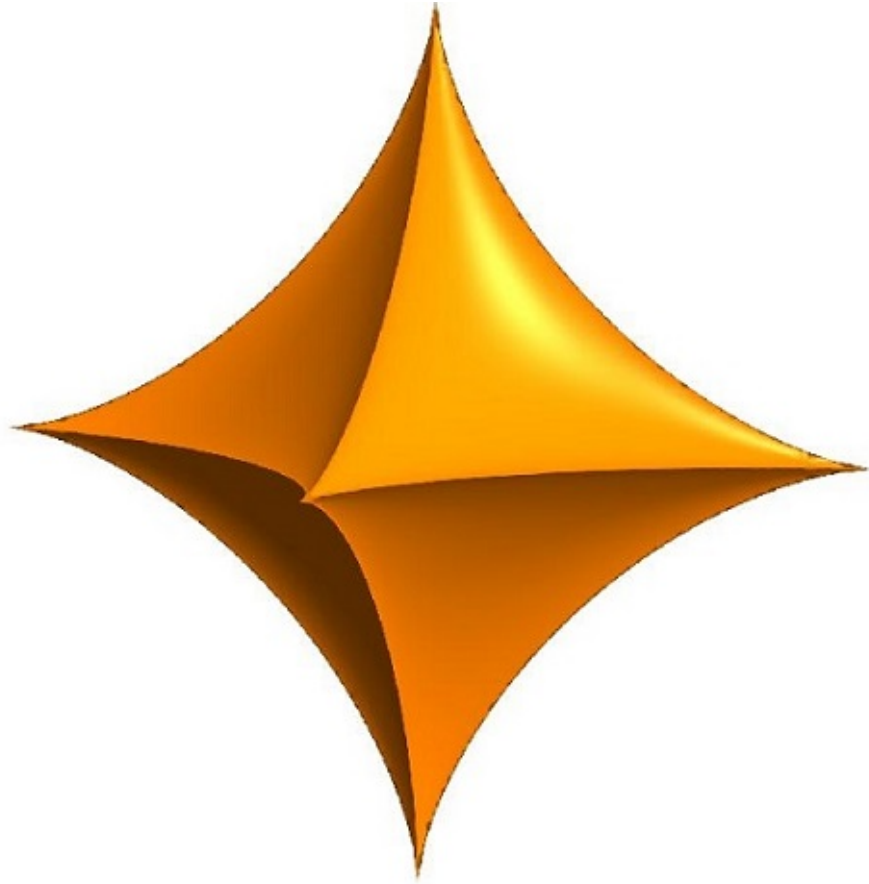
Obrázek 3.2: Trojrozměrná asteroida
