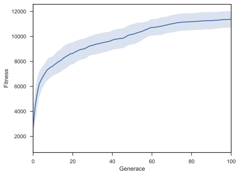
Obrázek 4.13: Mineral Worker chůze - průběh fitness DE
