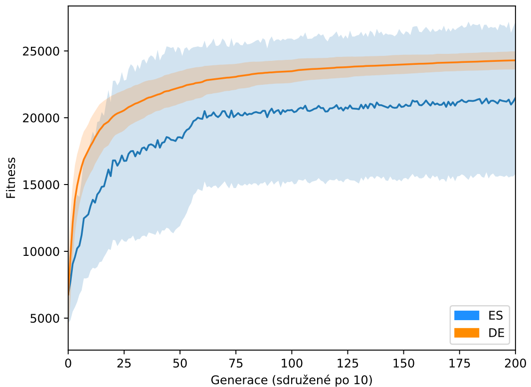
Obrázek 4.6: Wood Worker sbírání - porovnání průměrné fitness ES a DE
