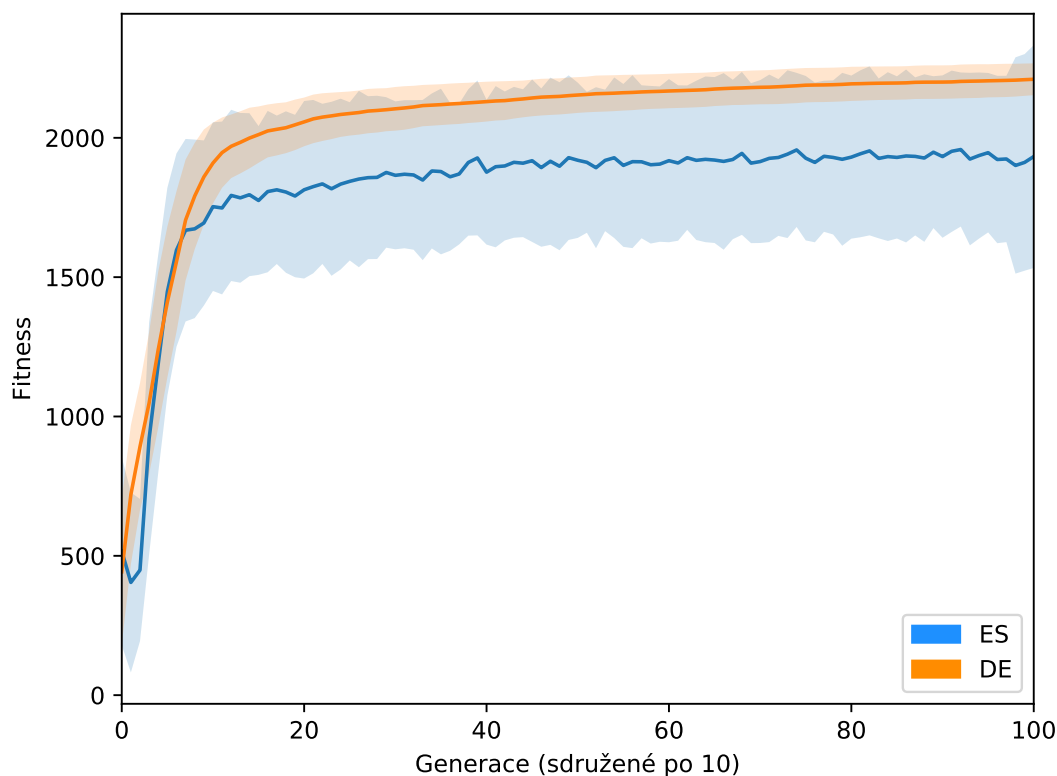
Obrázek 4.3: Wood Scout chůze - porovnání průměrné fitness ES a DE
