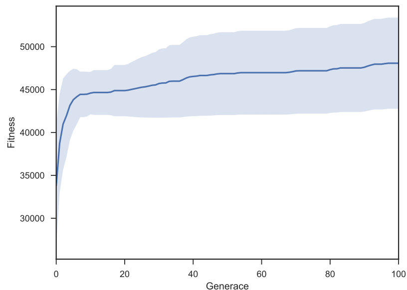
Obrázek 4.23: Competitive Scout agresivní - průběh fitness DE
