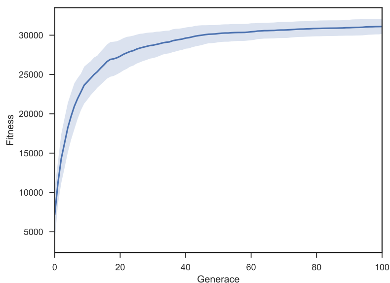
Obrázek 4.12: Mineral Scout chůze - průběh fitness DE
