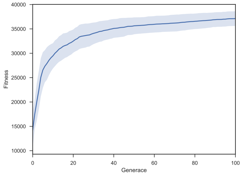
Obrázek 4.20: Competitive Scout chůze - průběh fitness DE
