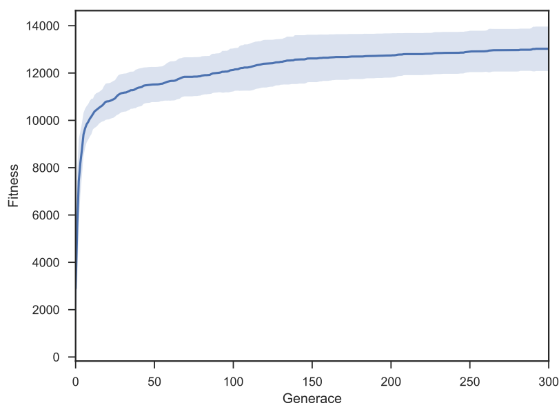
Obrázek 4.14: Mineral Worker sbírání - průběh fitness
