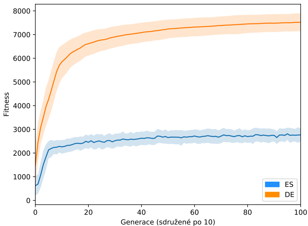
Obrázek 4.4: Wood Worker chůze - porovnání průměrné fitness ES a DE
