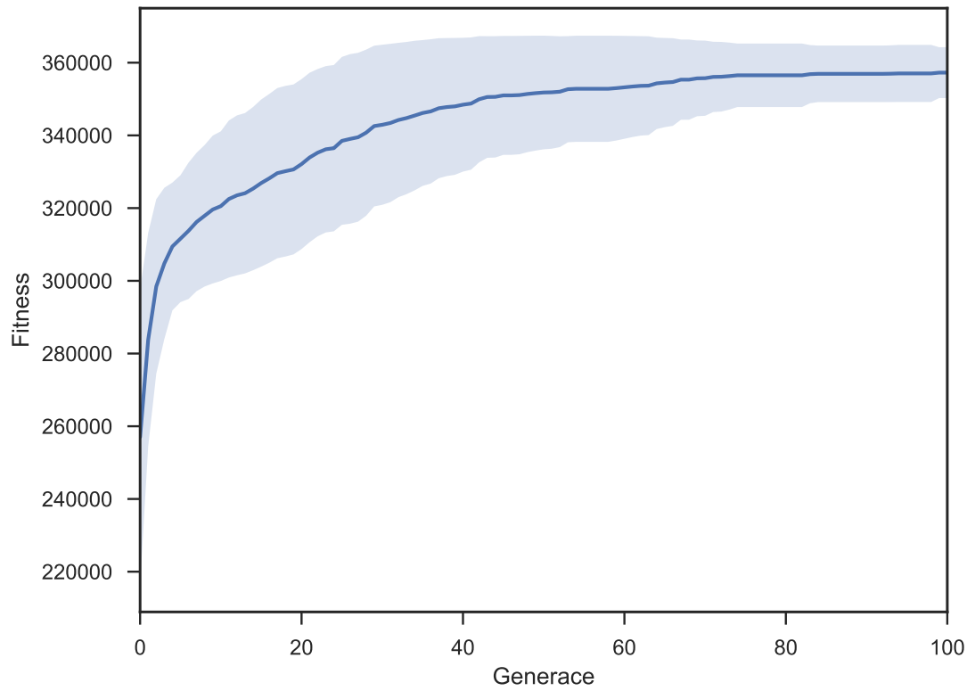
Obrázek 4.26: Competitive kooperace - průběh fitness DE
