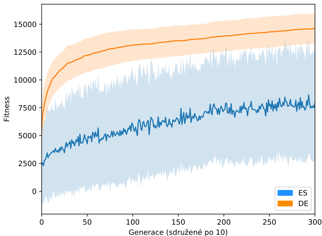
Obrázek 4.8: Wood hlavní úkol - porovnání průměrné fitness ES a DE
