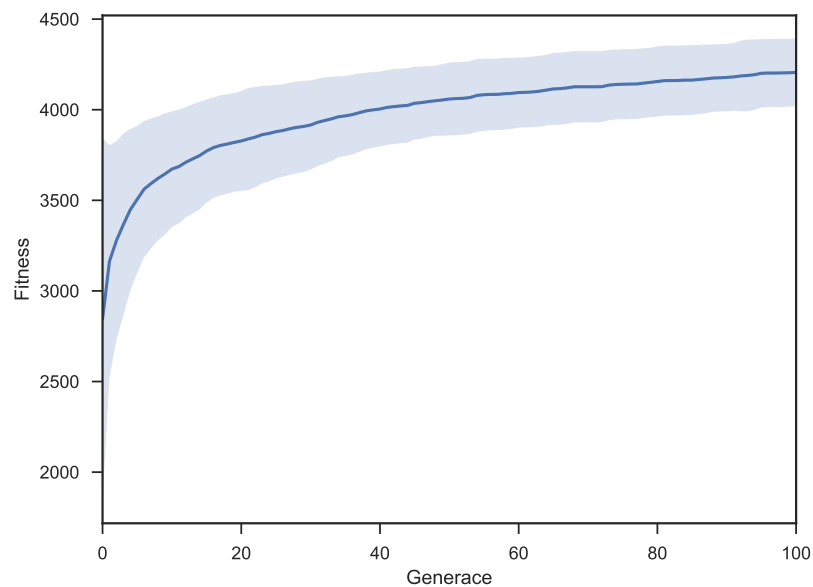
Obrázek 4.22: Competitive Scout životy - průběh fitness DE
