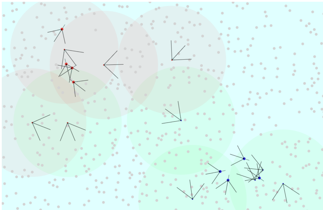
Obrázek 4.19: Příklad Competitive Scene mapy: start náhodného chování
