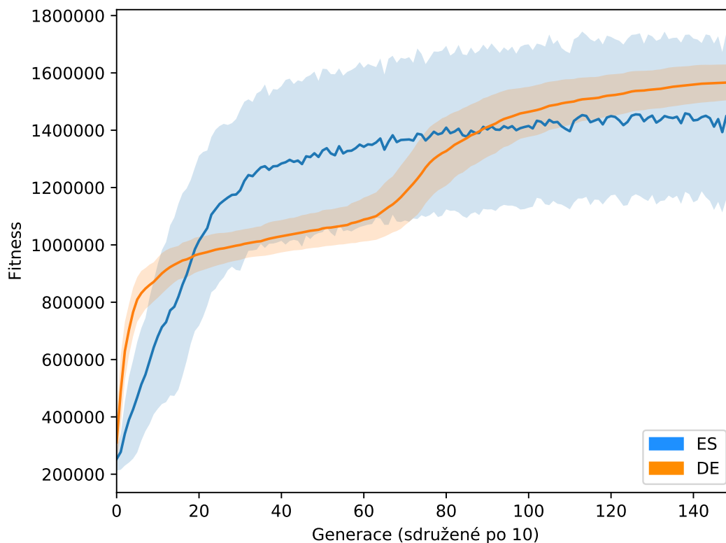
Obrázek 4.5: Wood Scout kácení - porovnání průměrné fitness ES a DE
