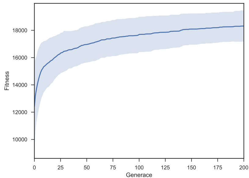
Obrázek 4.25: Competitive Fighter agresivní - průběh fitness DE
