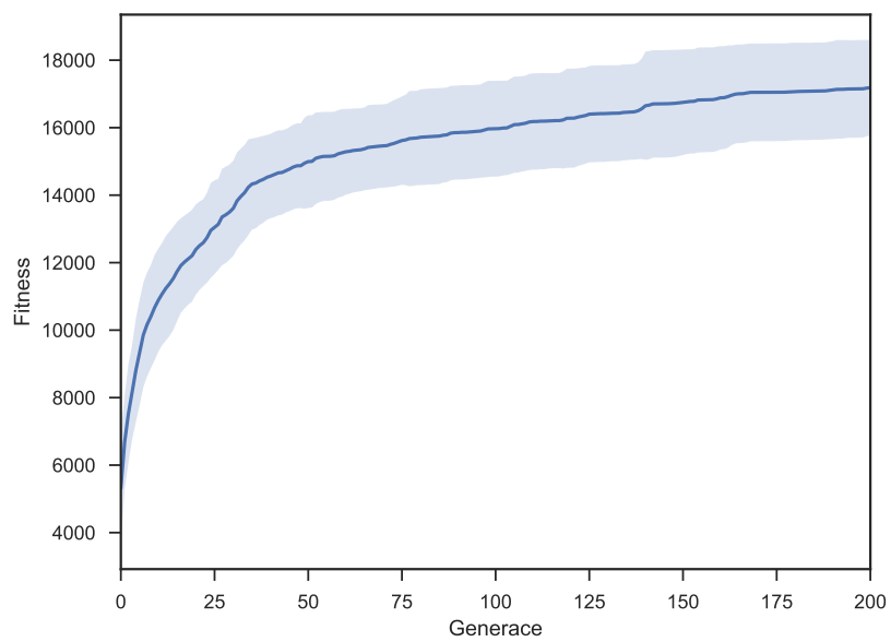
Obrázek 4.21: Competitive Fighter chůze - průběh fitness DE
