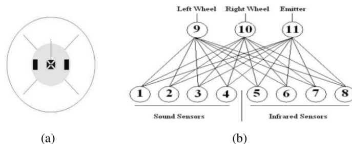
Obrázek 2.1: Cobot2D - nákres robota, Zdroj : (Yalcin, 2008)
