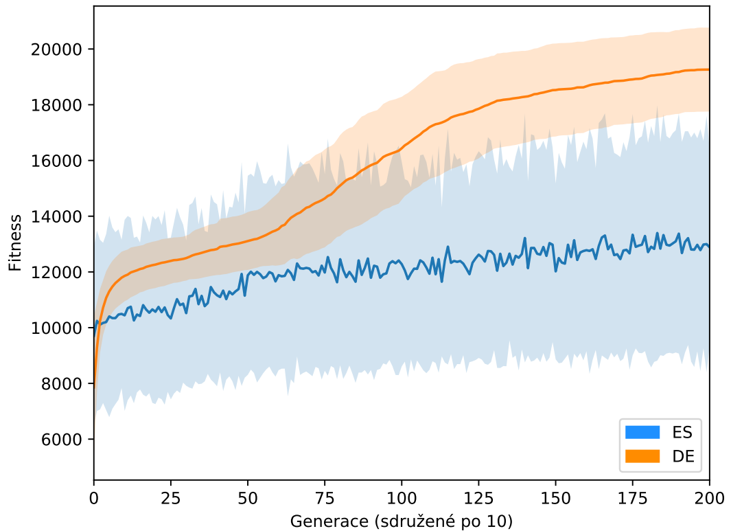
Obrázek 4.7: Wood Worker ukládání doprostřed - porovnání průměrné fitness ES a DE
