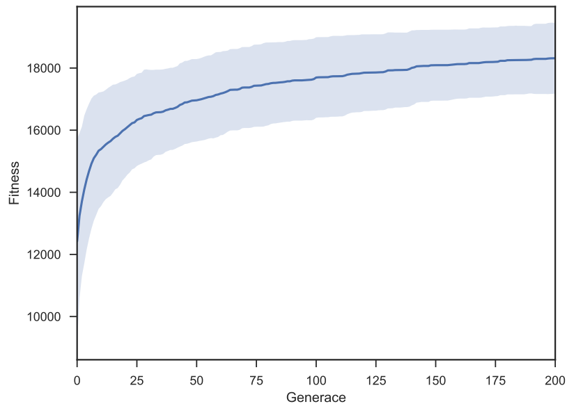
Obrázek 4.24: Competitive Fighter životy - průběh fitness DE
