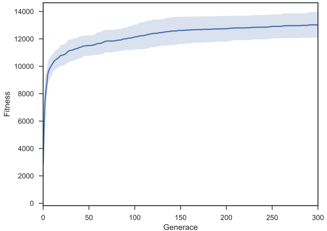
Obrázek 4.15: Mineral Worker skládání - průběh fitness DE
