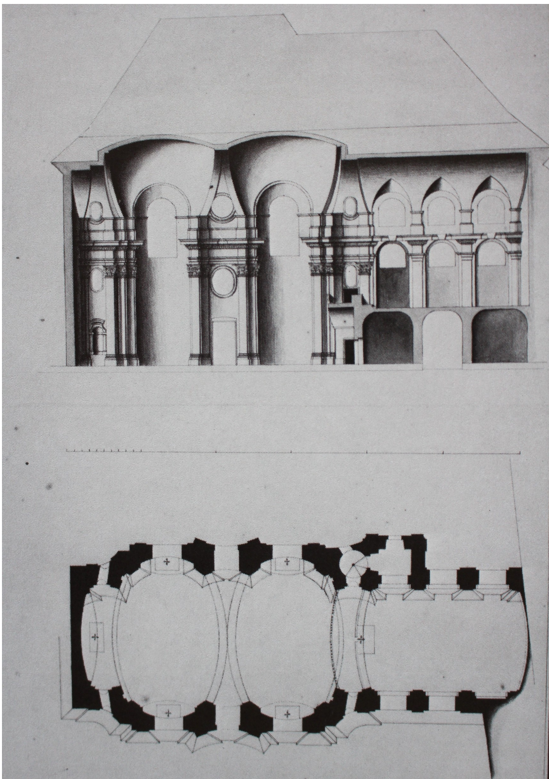
57. Cheb, kostel sv. Kláry, půdorys a podélný řez
