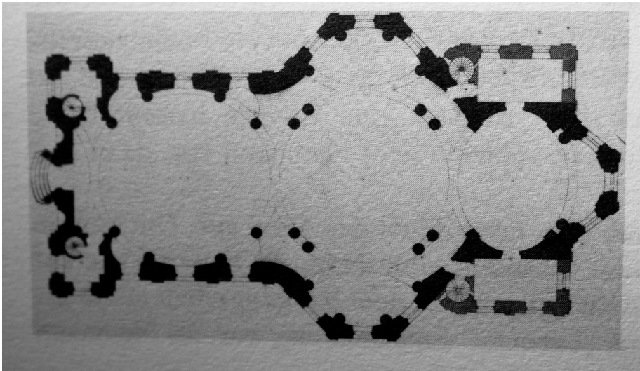
77. Vierzehnheiligen , bazilika Čtrnácti svatých pomocníků, půdorys- nerealizovaný návrh Balthasara Neumanna
