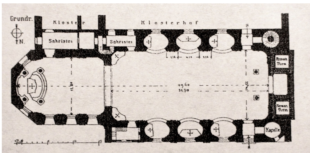
61. Osterhofen, klášterní kostel premonstrátů, půdorys
