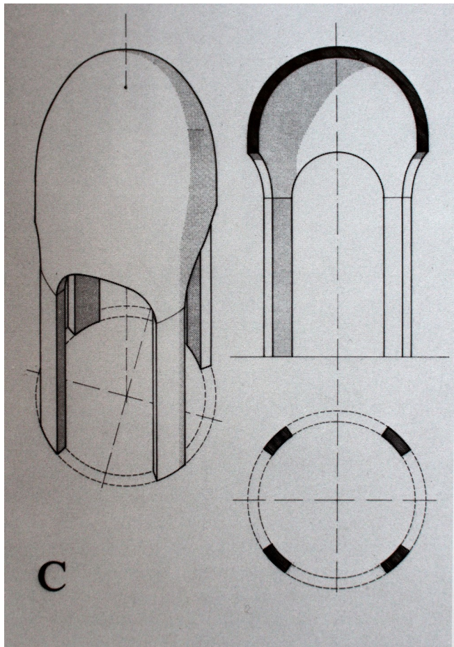
84. Schéma arkádové rotundy
