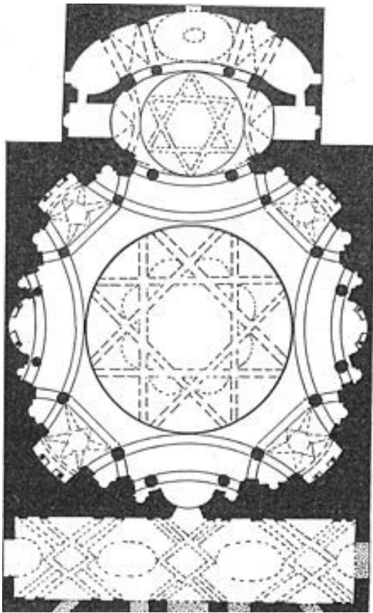
29. Turín , San Lorenzo, půdorys
