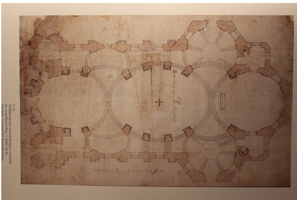
79. Vierzehnheiligen , bazilika Čtrnácti svatých pomocníků, půdorys
