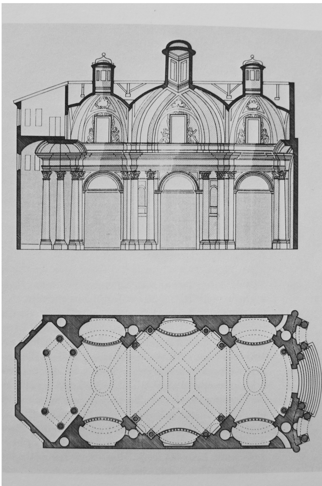
35. návrh na theatinský kostel v Praze, půdorys a řez
