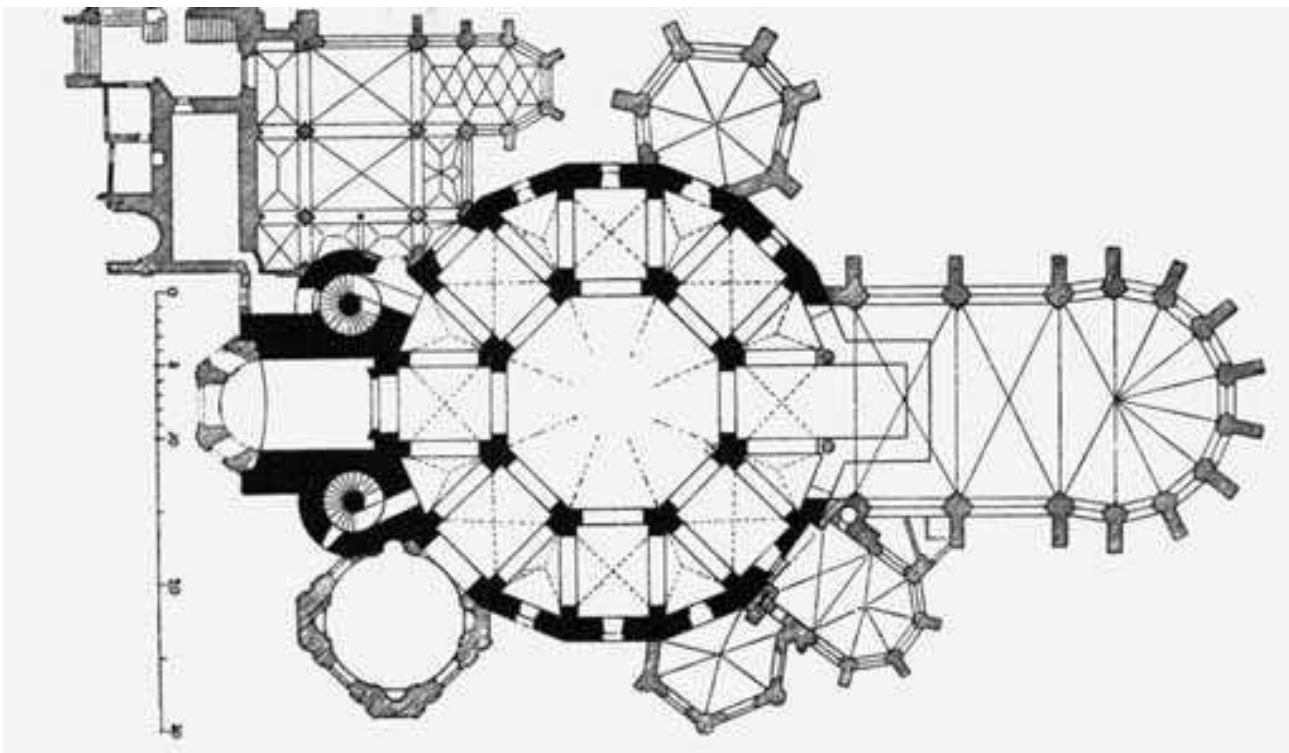
15. Cáchy, císařská kaple Karla Velikého v Cáchách, půdorys s gotickou přestavbou
