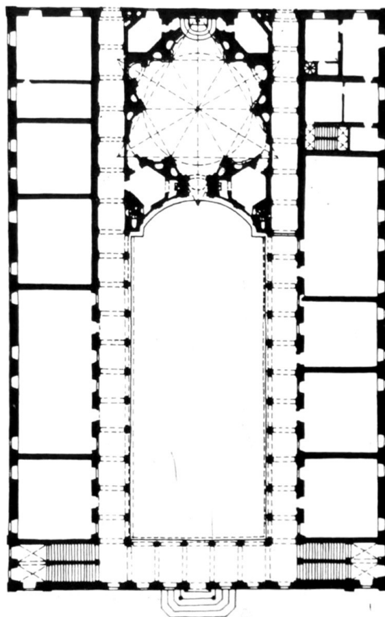
23. ŘÍM, Sant'Ivo alla Sapienza, půdorys kaple a půdorys zapojení areálu univerzity
