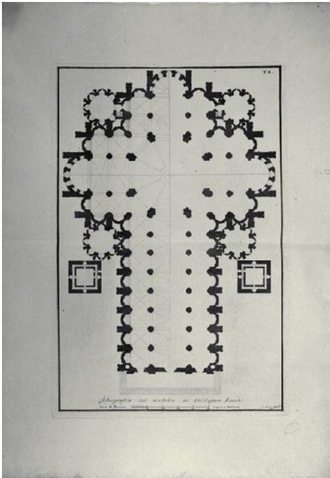
19. Pavia, Dóm v Pavii, půdorys dómu
