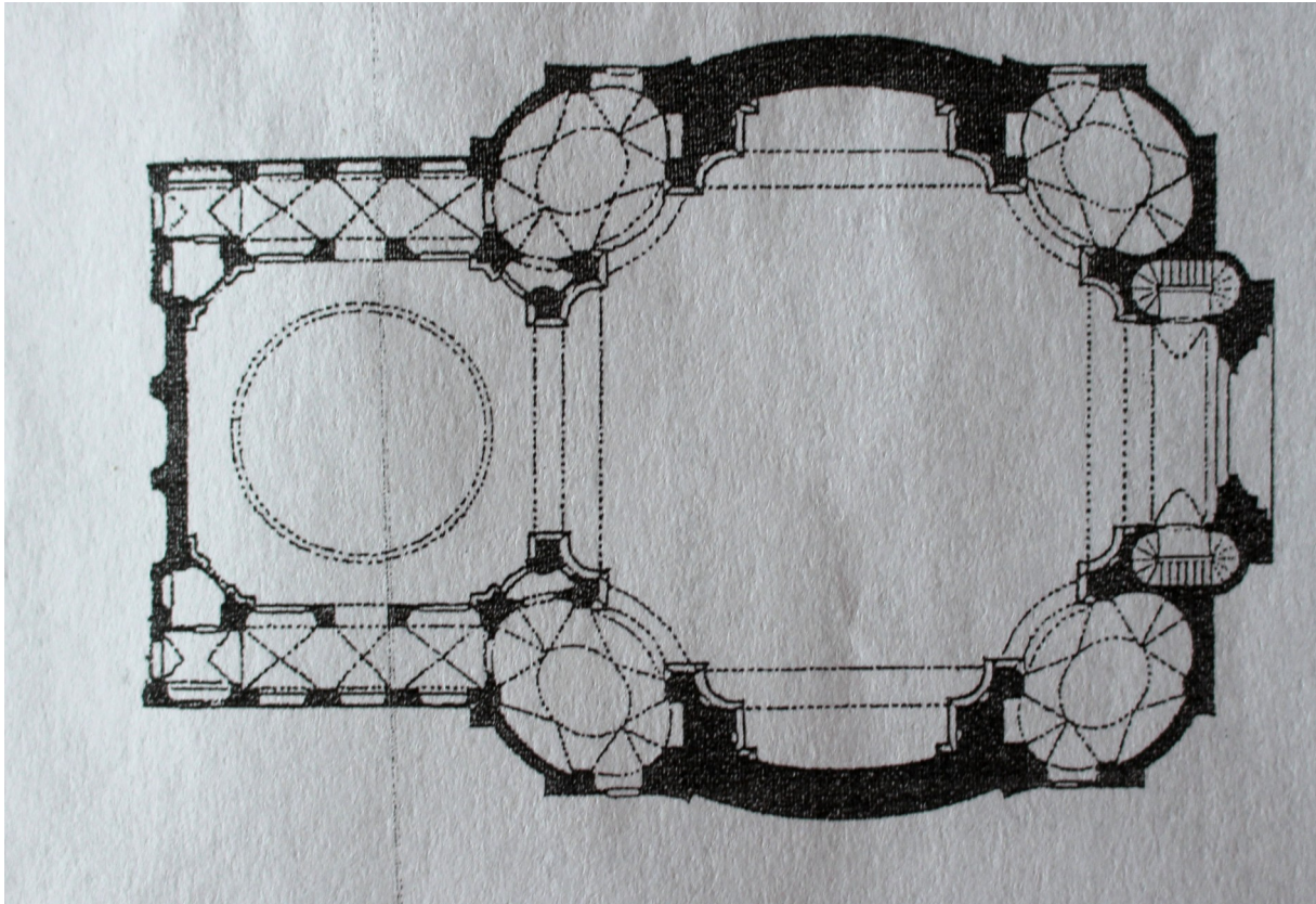
62. Ingolstadt, augustiniánský kostel, půdorys
