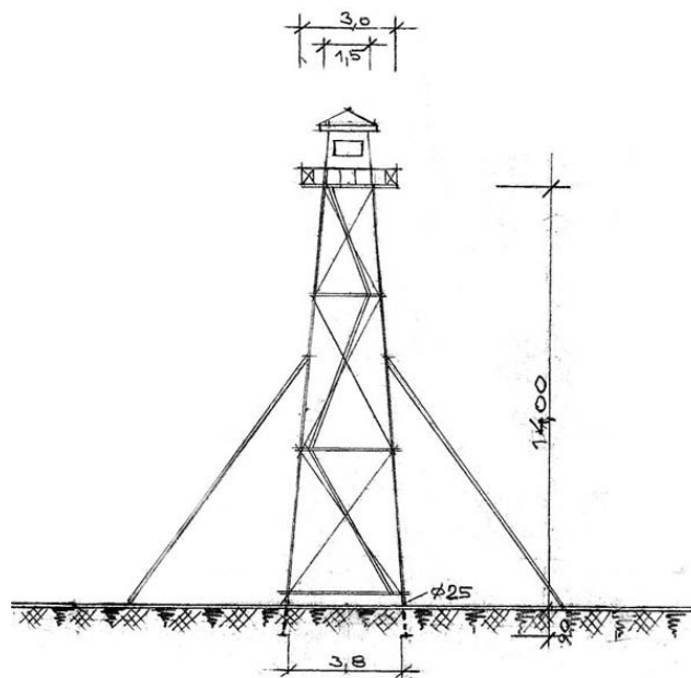
nákres věžové pozorovatelny.
