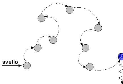
Obr. 3.6: Schéma koncentračného zhasínania luminiscencie. Absorbovaná energia je predávaná medzi luminiscenčnými centrami tvoriacimi reťazec pričom je nakoniec pohltená na centre nežiarivej rekombinácie, [30].
