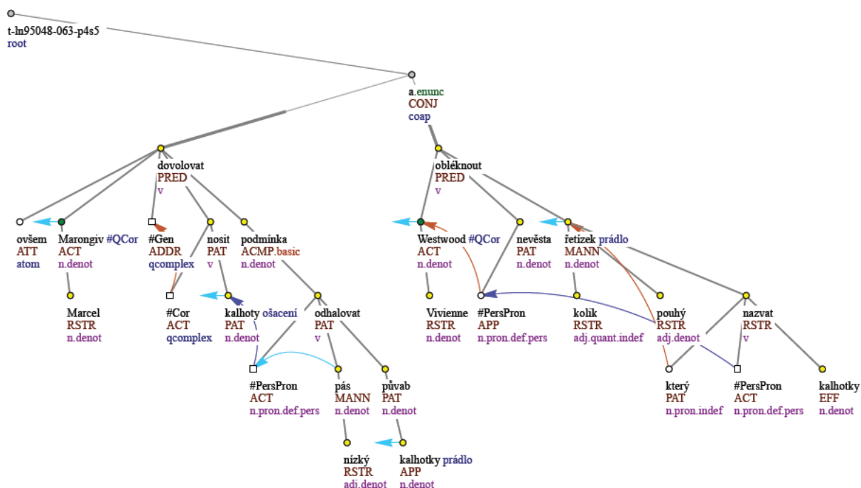
Obrázek 4: Příklad stromu z PDT obsahujícího altlex s funktorem ACMP
