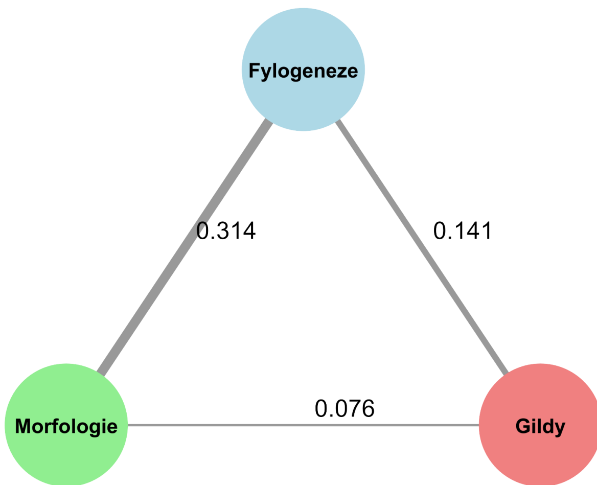
Obr. 14: Vizualizace korelací mezi morfologií, potravním chováním (gildy) a fylogenezí v datasetu australských pěvců. Čísla značí míru korelace pomocí Mantelova r .
