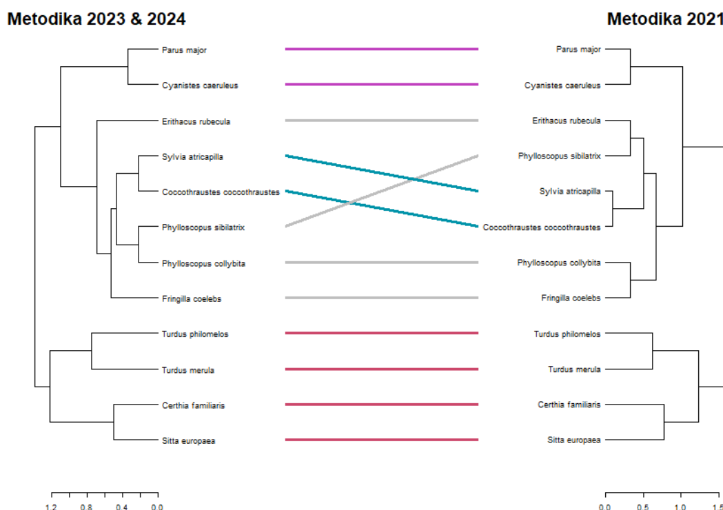
Obr. 8: Kodendrogram gild v NPR Koda pro porovnání výsledků mezi lety 2021 a 2023 & 2024. Barevné čáry značí stejnou topologii dendrogramu na obou stranách, šedivé značí odlišnosti. Měřítka pod dendrogramy značí Bray-Curtisovu vzdálenost.
