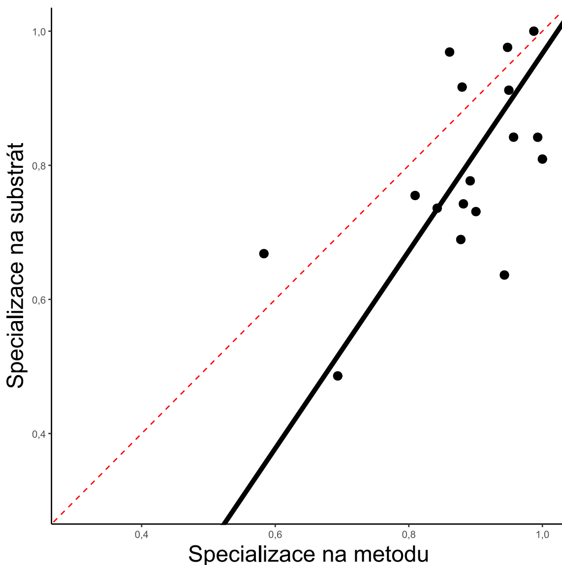
Obr. 5: Graf specializace na metodu a substrát. Osy x a y byly omezeny na škálu 0,4–1 pro lepší čitelnost, neboť žádný druh nižších hodnot nedosahuje. Pomocná červená šrafovaná přímka má sklon = 1 a dělí graf diagonálně. Černou barvou je vyznačena úsečka regrese typ II (RMA), která zobrazuje vztah mezi body.
