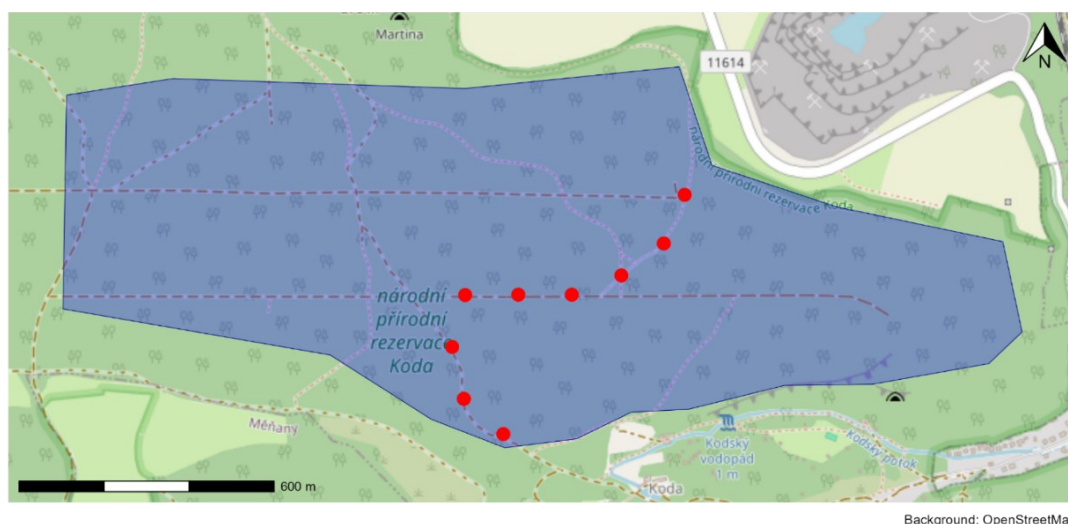
Obr. 2: Mapa lokality s modře vyznačeným areálem pro sběr dat a s červenými tečkami bodového transektu.
