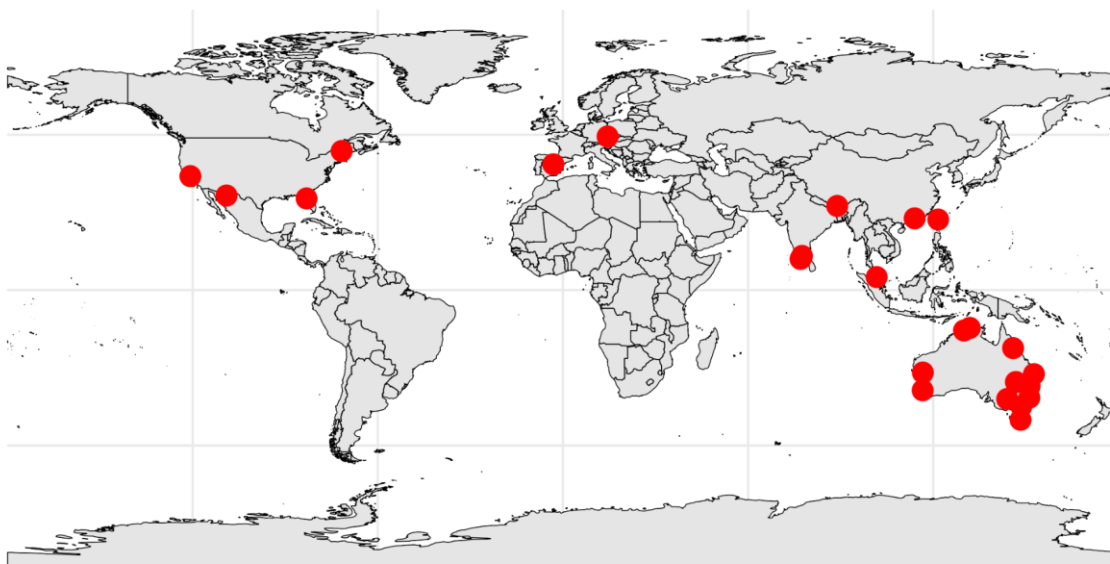
Obr. 9: Mapa světa s lokacemi zdrojů dat pro mezikontinentální srovnání. Každá červená tečka značí jednu práci. Poloha je přibližná, přesné údaje jsou k dohledání v jednotlivých pracích.
