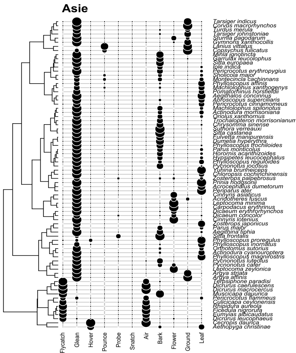
Obr. 19: Vizualizace využívaných substrátů a metod pro dataset 75 druhů asijských pěvců. Dendrogram značí shluky dle potravního chování, velikost černých kruhů je úměrná proporci využívání dané metody/substrátu druhem.
