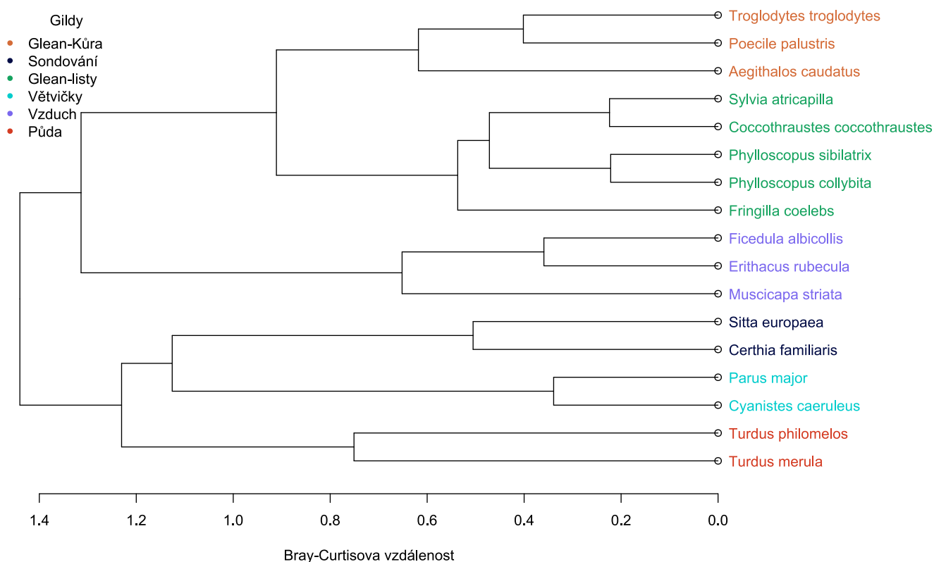
Obr. 6: Dendrogram znázorňující gildy pěvců založené na shlukování distanční matice Bray-Curtis vzdáleností dle využívání potravních substrátů a metod. Barevně vyznačené gildy jsou pojmenovány podle vlastností, které nejlépe charakterizují dané skupiny.
