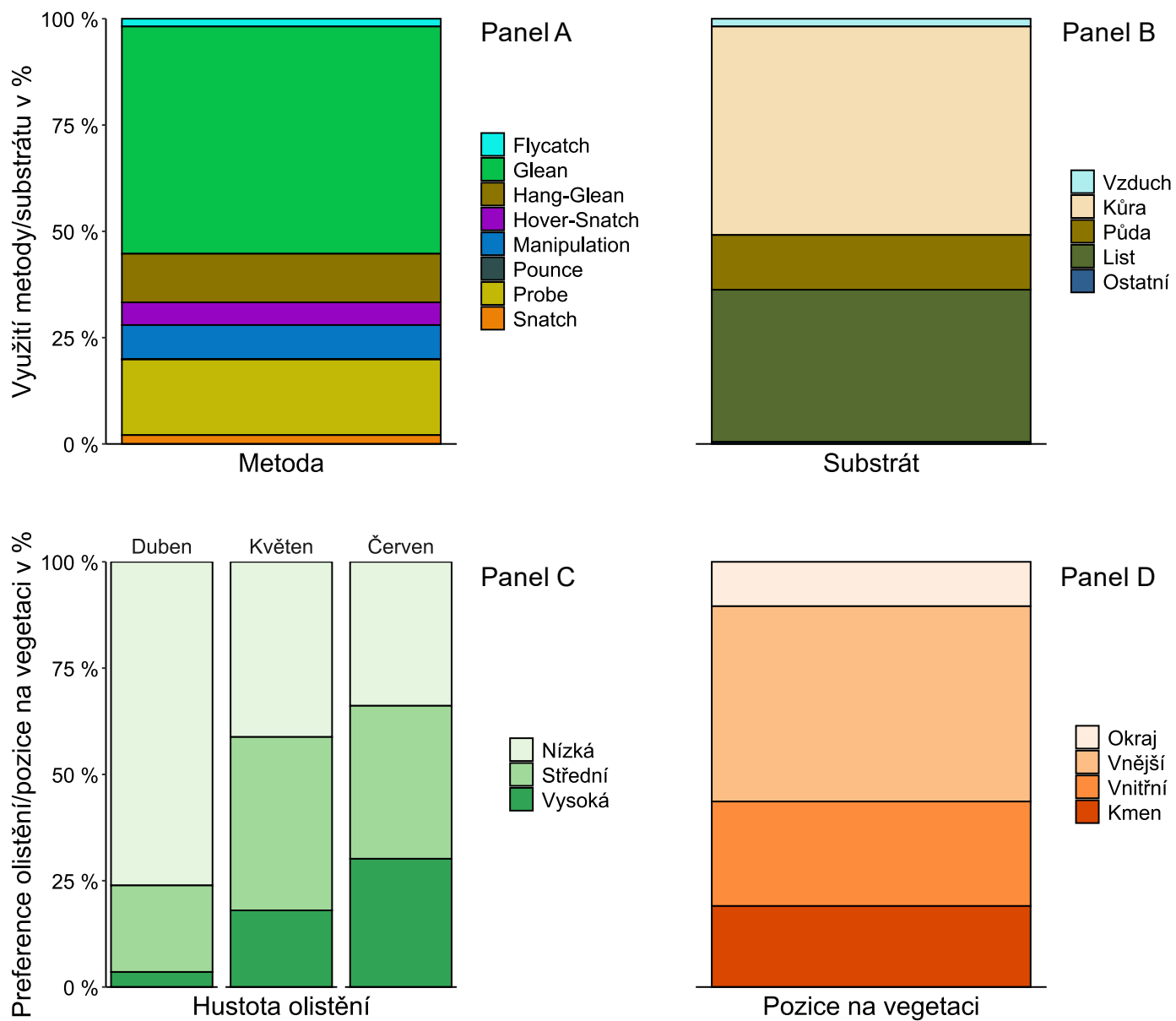
Obr. 4: Frekvence využití metod a substrátů (panely A a B) a preference olistění a pozice na stromě (panely C a D) pro sběr potravy 17 druhů pěvců ( n = 2790 potravních událostí). Graf hustoty olistění je zobrazen pro každý měsíc zvlášť.
