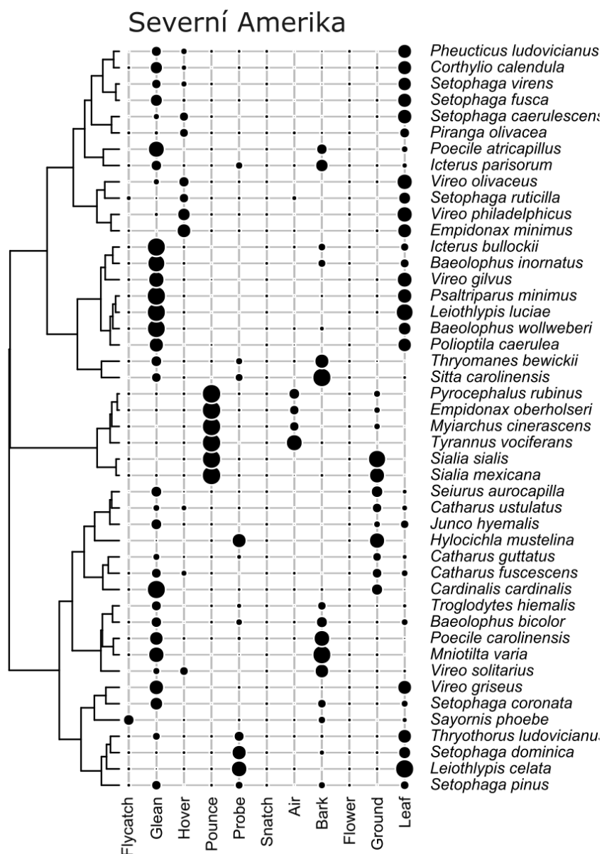
Obr. 22: Vizualizace využívaných substrátů a metod pro dataset 46 druhů severoamerických pěvců. Dendrogram značí shluky na základě potravního chování, velikost černých kruhů je úměrná proporci využívání dané metody/substrátu druhem.
