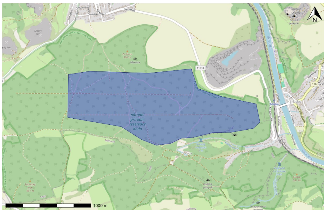
Obr. 1: Mapa okolí lokality s přibližným areálem pro sběr dat vyznačeným modrým mnohoúhelníkem. Plocha pro vzorkování činila asi 1,4 km 2 .
