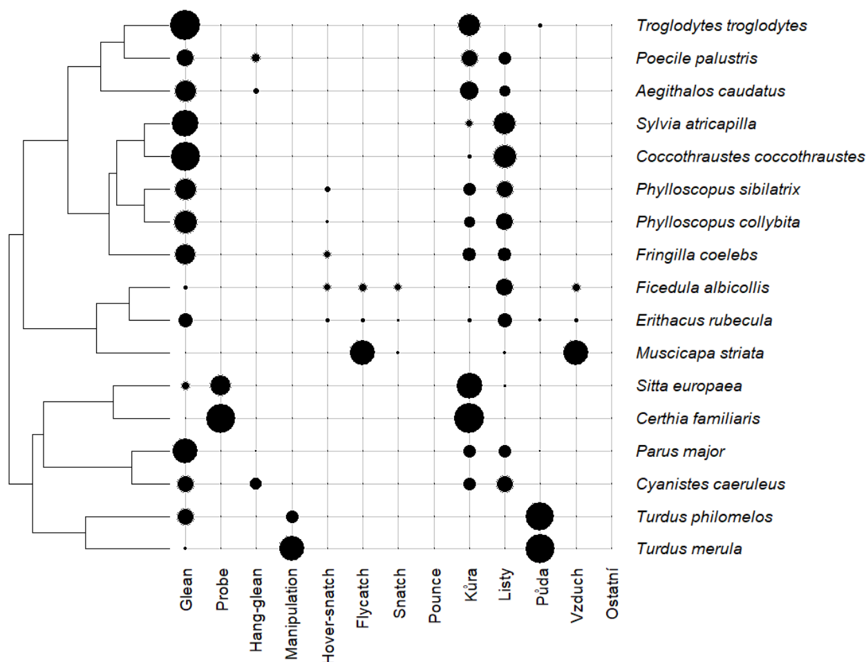
Obr.7: Proporce využívání metod a substrátů jednotlivých druhů v trofických gildách. Velikost černých kruhů značí proporce využití metody či substrátu pro daný druh. Dendrogram na levé straně je tentýž jako při zobrazení gild na obr.6.
