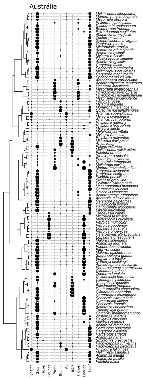
Obr. 16: Vizualizace využívaných substrátů a metod pro dataset 115 druhů australských pěvců. Dendrogram značí shluky dle potravního chování (gildy), velikost černých kruhů je úměrná proporci využívání dané metody/substrátu druhem. Graf jako vektorový soubor viz repozitář.
