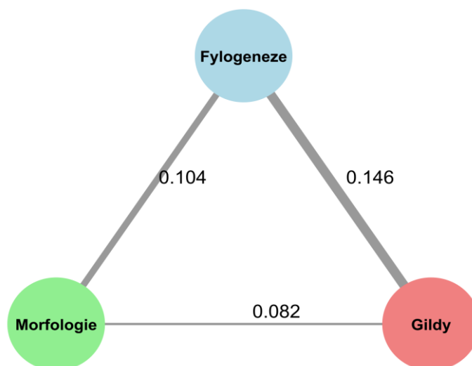
Obr.10: Vizualizace korelací mezi fylogenezí, morfologií a potravním chováním (gildy). Číslo značí míru korelace pomocí Mantelova r.
