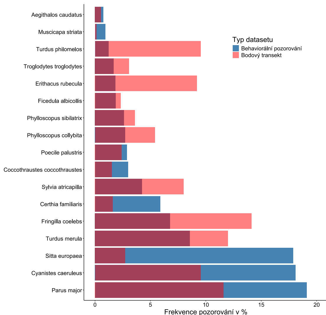
Obr. 3: Histogram zobrazující rozdíly ve frekvencích pozorování podmnžiny druhů na bodovém transektu (červeně) a při sběru dat o potravním chování (modře).
