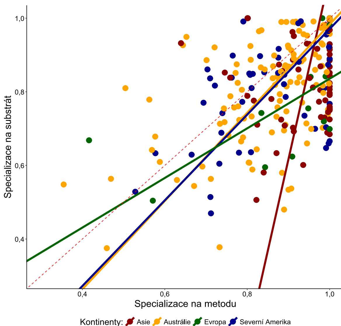
Obr. 13: Graf zobrazující hodnoty indexu specializace na substrát a metodu. Každý bod představuje jeden druh, barevně označený dle kontinentu (viz legenda). Červená přerušovaná čára se sklonem = 1 dělí graf diagonálně pro přehlednost. Barevné úsečky jsou produktem regrese model II (RMA) a zobrazují vztah mezi specializací na metodu a substrát druhů daného kontinentu.
