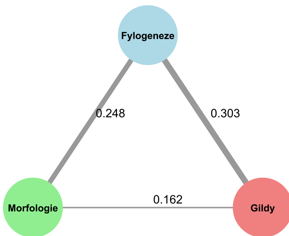
Obr. 17: Vizualizace korelací mezi morfologií, potravním chováním (gildy) a fylogenezí v datasetu asijských pěvců. Čísla značí míru korelace pomocí Mantelova r .
