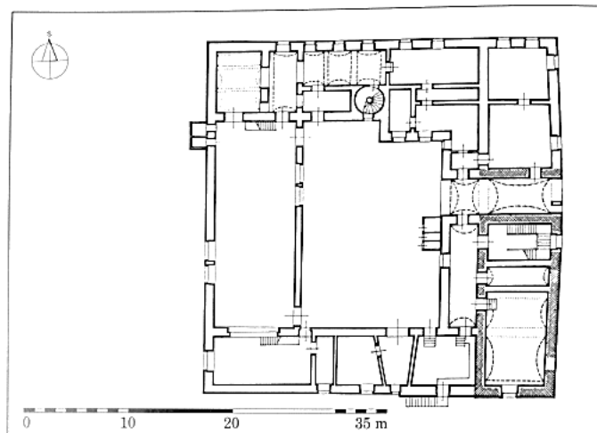
Obr. 244: Štítina. Půdorysné zaměření s vyznačením nejstarší fáze v úrovni přízemí.
