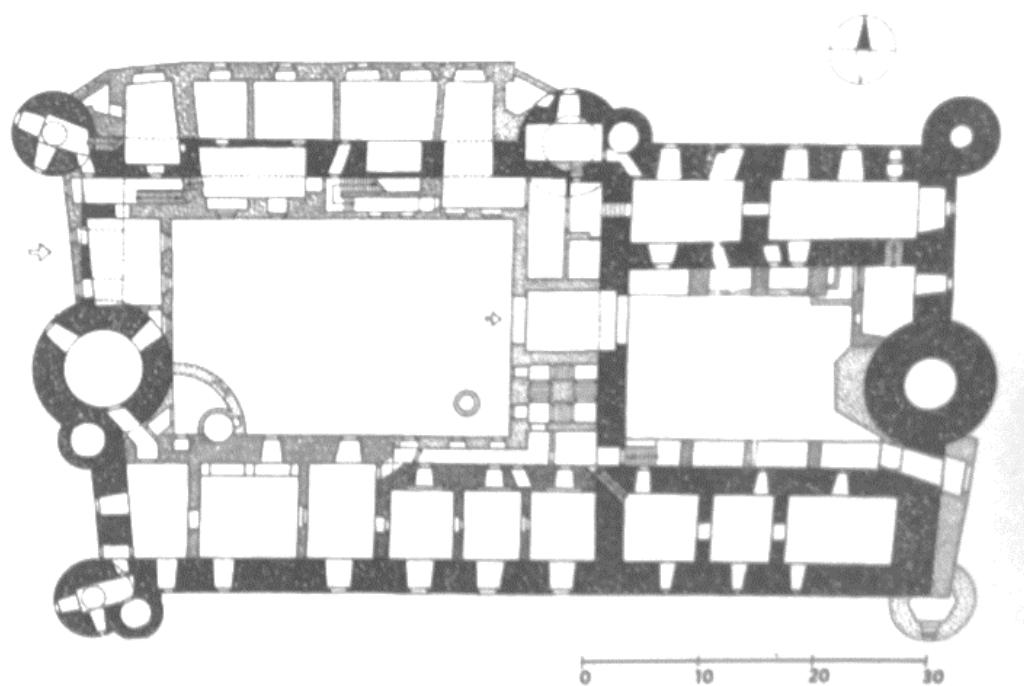
440 KONOPIŠTĚ, přízemí hradu. Zrněné zdivo z počátku 14. stol., křížkované z počátku 16., šrafované ze začátku 17. a tečkované z 18. stol. a pozdější.
