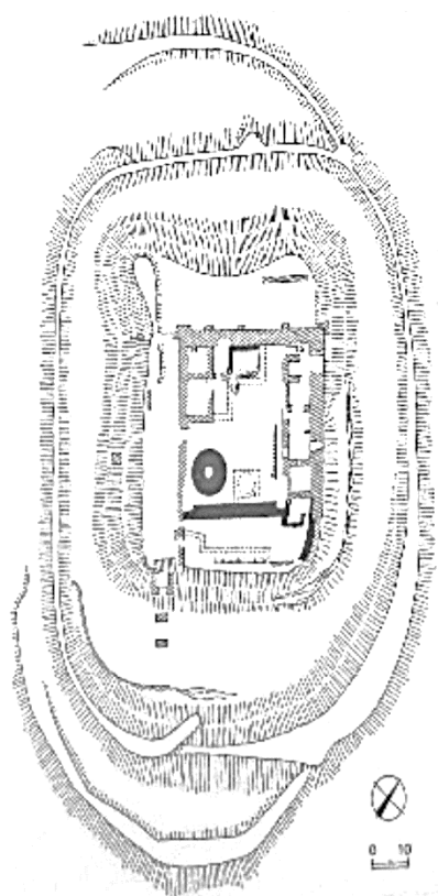
Cvilín. Půdorys hradu se složitější zástavbou a pravidelným obrysem. Černě pozůstatky z doby okolo poloviny 13. století, šrafované přestavba z 15.–16. století. Čarkované jsou doplněna zdiva z předválečných výkopů.
