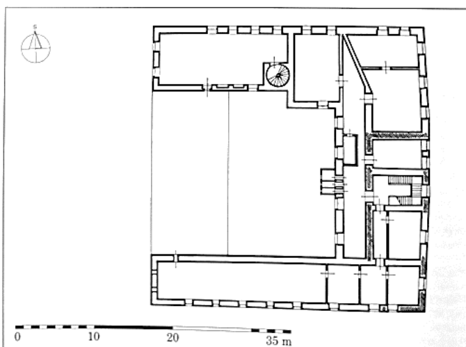
Obr. 245: Štítina. Půdorysné zaměření s vyznačením nejstarší fáze v úrovni 1. patra.
