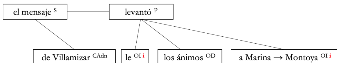
Graf 2: Návrh na syntaktickou analýzu věty <10>
