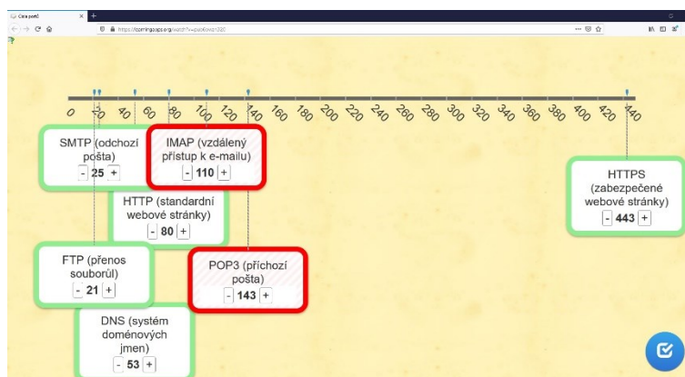
Obrázek 12 Číselná osa v aplikaci LearningApps (snímek obrazovky)
